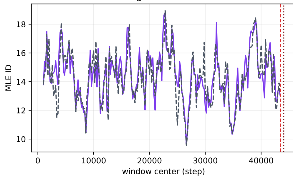
grad cosine
