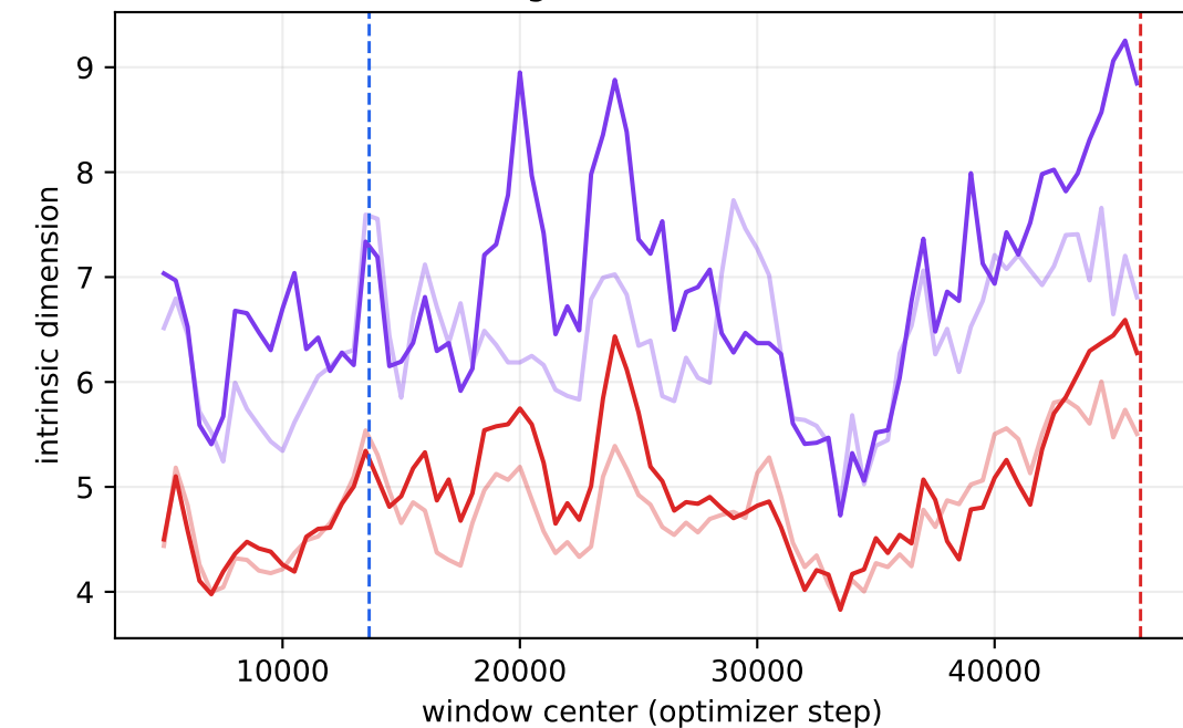
gradient norm
