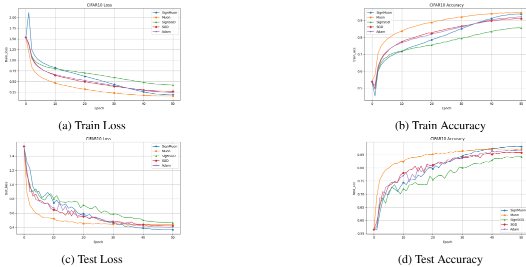
Рис. 2: Сравнение сходимости и точности различных алгоритмов оптимизации на обучении классификатора CIFAR-10.
