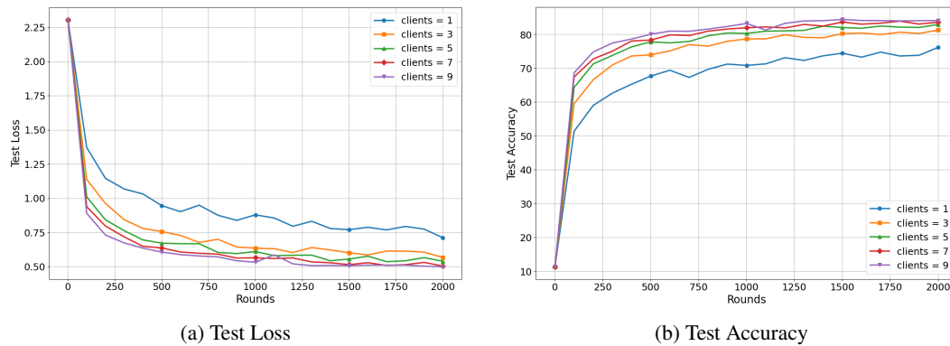
Рис. 6: Федеративное обучение. Эксперимент 1. Масштабируемость алгоритма SignMuon.
