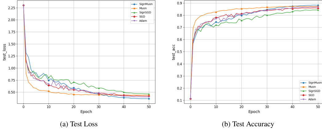
Рис. 5: Централизованный сценарий. Сравнение сходимости и точности различных алгоритмов оптимизации на обучении классификатора CIFAR-10 на тестовой выборке.
