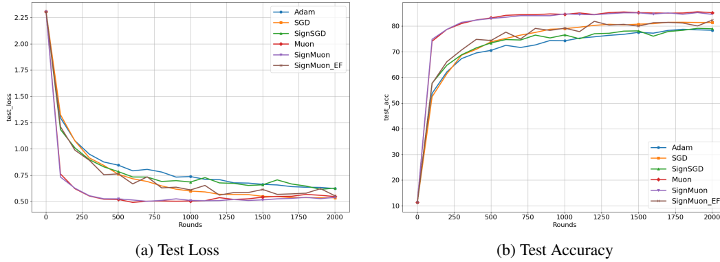
Рис. 8: Федеративное обучение. Эксперимент 3. Сравнение разных алгоритмов при числе клиентов n=10 .
