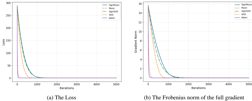
Рис. 1: Гладкая выпуклая задача (уравнение 27) для матрицы 500 \times 500 .
