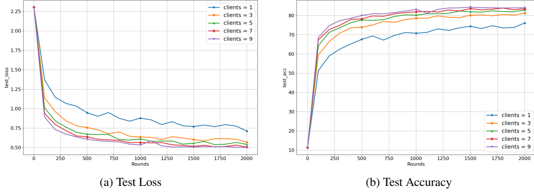
Рис. 6: Федеративное обучение. Эксперимент 1. Масштабируемость алгоритма SignMuon.
