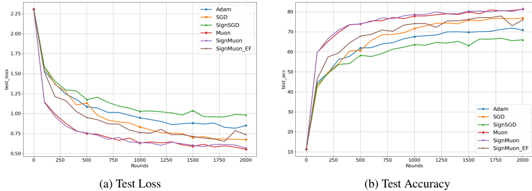
Рис. 7: Федеративное обучение. Эксперимент 2. Сравнение разных алгоритмов при числе клиентов n=3 .
