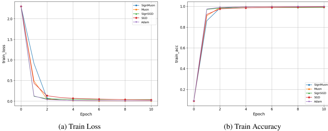
Рис. 1: Сравнение сходимости и точности различных алгоритмов оптимизации на обучении классификатора MNIST на тренировочной выборке.
