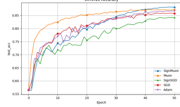
(d) Test Accuracy
