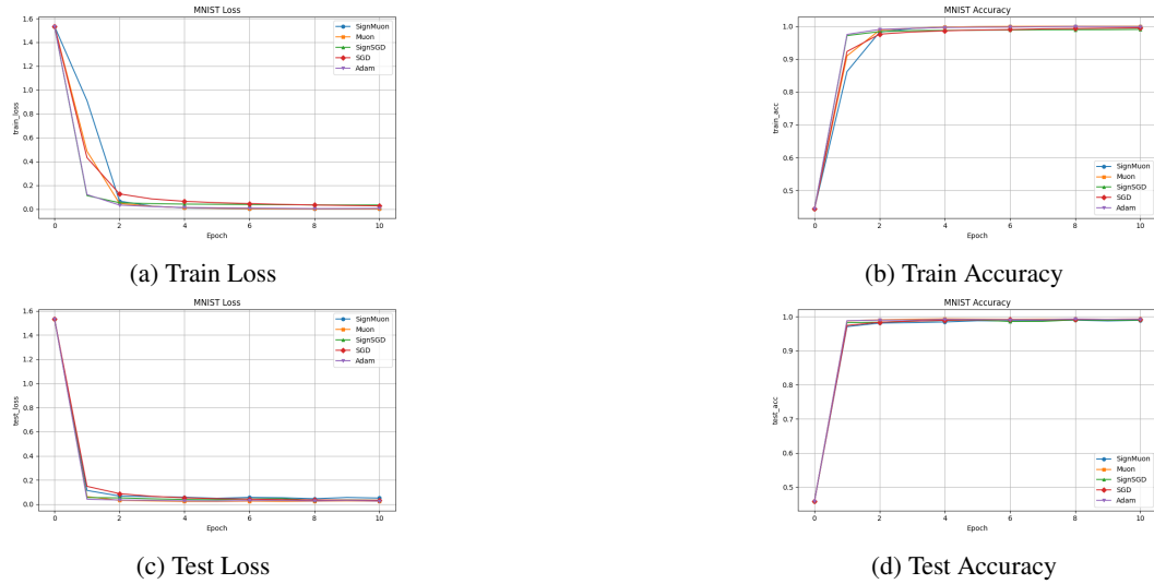
Рис. 1: Сравнение сходимости и точности различных алгоритмов оптимизации на обучении классификатора MNIST.
