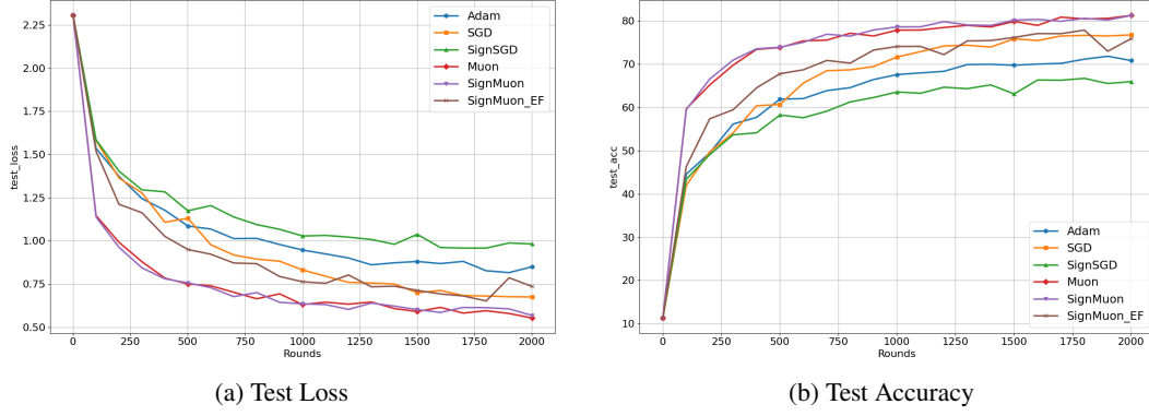
Рис. 6: Федеративный сценарий. Эксперимент 2. Сравнение разных алгоритмов при числе клиентов p=3 .
