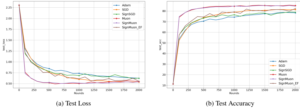
Рис. 7: Федеративный сценарий. Эксперимент 3. Сравнение разных алгоритмов при числе клиентов p=10 .
