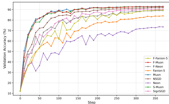
Точность на валидационной выборке
