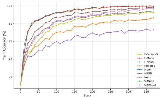
Точность на обучающей выборке
