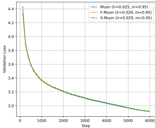
Модель GPT-2 Medium
