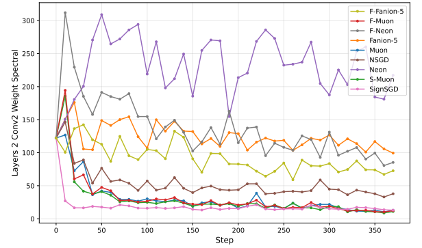
(d) Spectral norm of layer2.conv2
