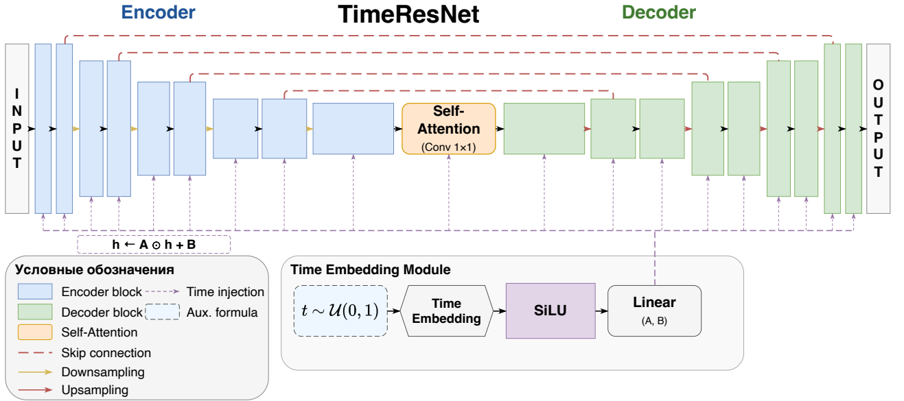
Рис. 2: Архитектура TimeResNet: U-Net с поблочной аффинной временной модуляцией и модулем самовнимания на буттлнеке. Единственная сеть используется для обоих направлений трансляции.
