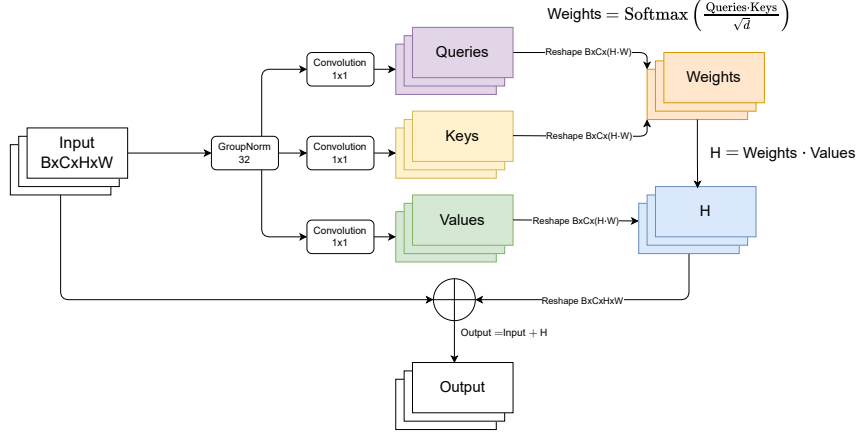
Рис. 4: Модуль свёрточного self-attention на бутлнеке: GroupNorm \rightarrow 1 \times 1 Conv ( Q, K, V ) \rightarrow развёртывание \rightarrow масштабированное скалярное произведение (29)–(30) \rightarrow остаточное сложение (31).
