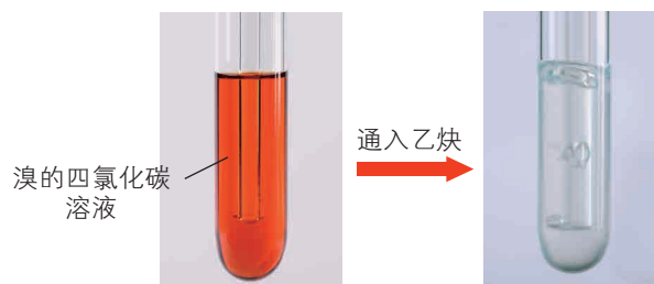
图1-3-6 乙炔与溴的四氯化碳溶液的反应
