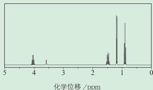
图1-4-5 分子式为 \text{C}_4\text{H}_{10}\text{O} 的有机化合物X的核磁共振氢谱图
