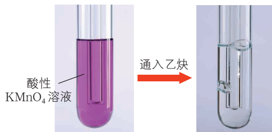
图1-3-7 乙炔与酸性KMnO 4 溶液的反应
