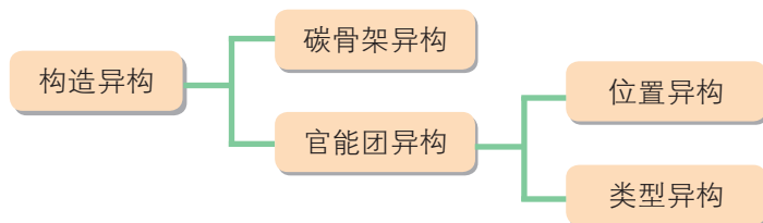
图1-2-8 构造异构的表现形式示意图
