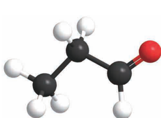
丙醛 ( \text{CH}_3\text{CH}_2\text{CHO} )
