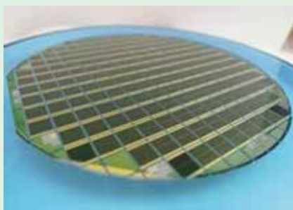
图1-5-5 砷化镓太阳电池
