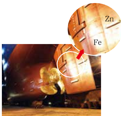
图1-4-4 用牺牲阳极保护法保护金属船体和铁管道
