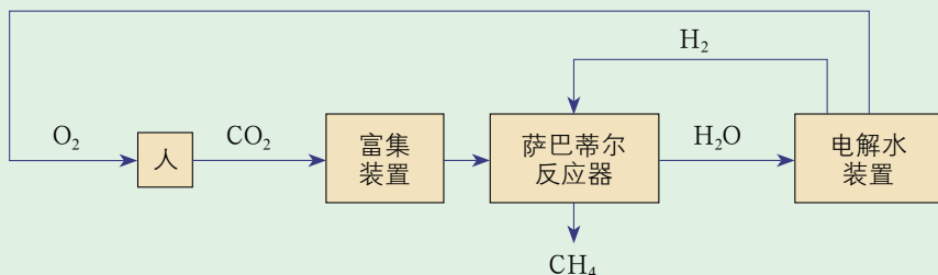
图1-5-6 利用萨巴蒂尔反应的氧气再生方法
