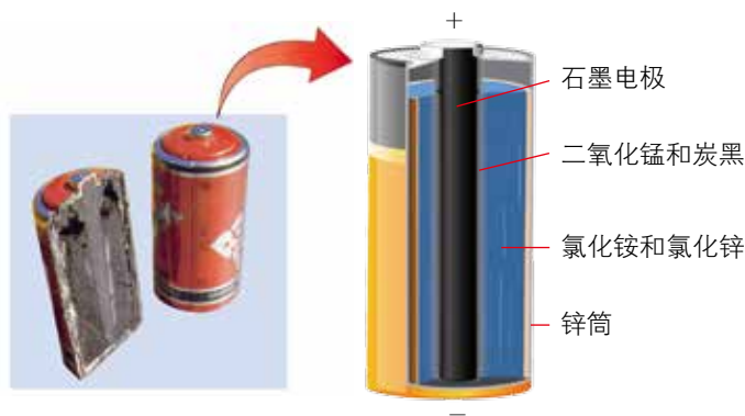
图1-2-5 酸性锌锰干电池及其结构示意图
