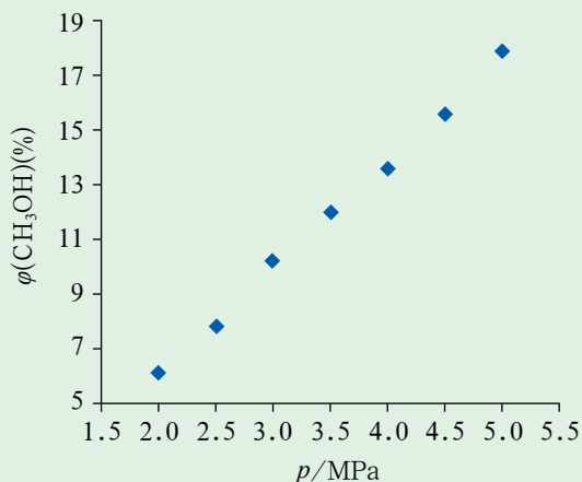
图2-5-1 不同总压对甲醇产率的影响
