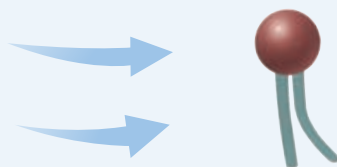
磷脂分子示意图
