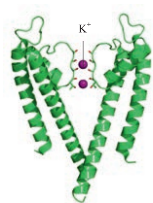
▲ 图 4-5 钾离子通道模式图
