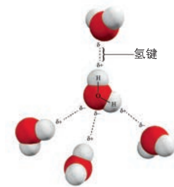
水分子之间靠氢键结合示意图
