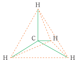
图3-1-5 甲烷分子的空间结构示意图
