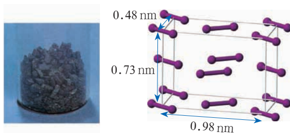
图3-2-12 碘晶体及其晶体结构
