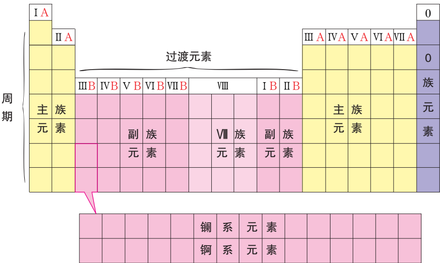
图1-2-5 元素周期表轮廓图
