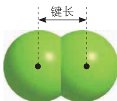
图2-1-9 氯分子中 Cl—Cl 键的键长
