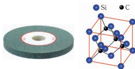
图3-2-10 碳化硅砂轮及碳化硅晶体结构
