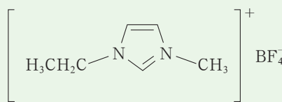
图3-2-7 1-乙基-3-甲基咪唑 四氟硼酸盐的结构
