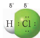
H—Cl
