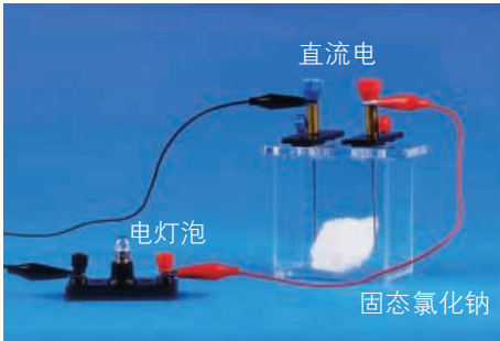
固态氯化钠不能导电
