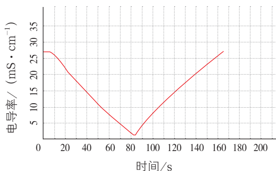
图 2-2-8 关于稀硫酸与 \text{Ba}(\text{OH})_2 溶液反应实质的研究
