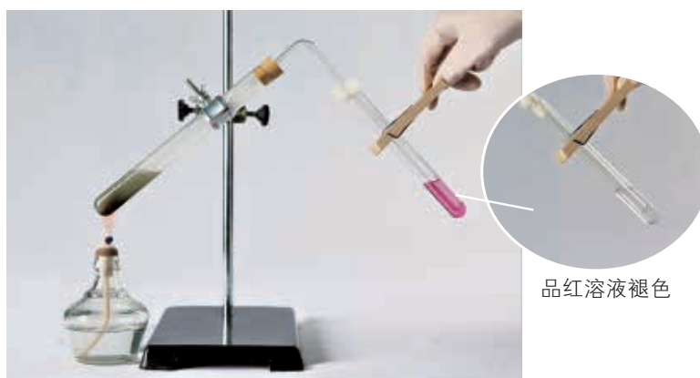
图 3-2-10 浓硫酸与铜反应的实验
