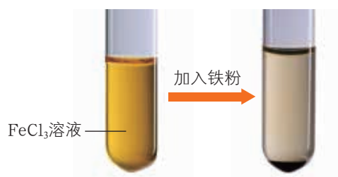
图 3-1-3 \text{FeCl}_3 溶液与铁粉的反应
