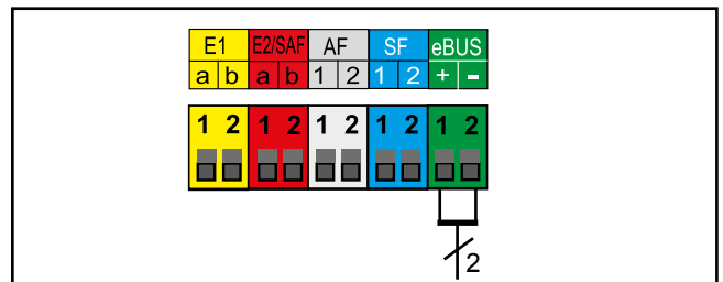
Bild: Anschluss Wolf-Regelungszubehör digital (eBus-Schnittstelle)
