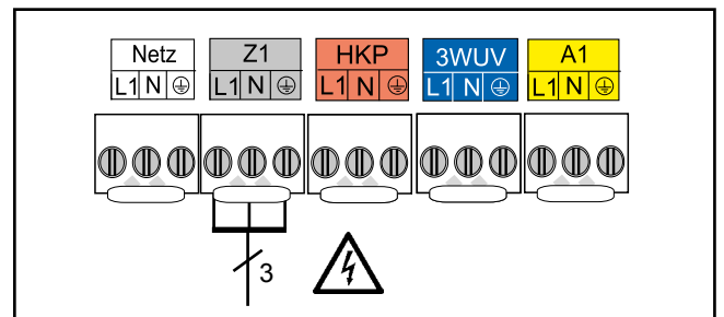
Bild: Anschluss Ausgang Z1
