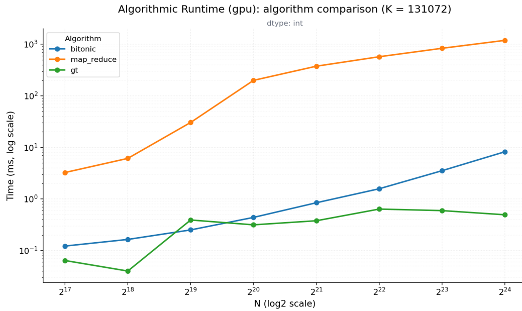
Σχήμα 7.5: Οι τρεις αλγόριθμοι στη μονάδα γραφικών για k ίσο με 131072.
