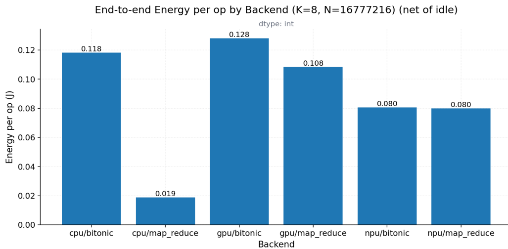
Σχήμα 7.12: Καθαρή ενέργεια ανά αρχιτεκτονική και αλγόριθμο, για k ίσο με 8.
