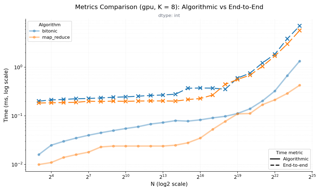
Σχήμα 7.11: Αλγοριθμικός και συνολικός χρόνος στη μονάδα γραφικών, για κ ίσο με 8. Η απόσταση των δύο καμπυλών κάθε αλγορίθμου είναι το κόστος των μεταφορών και της έναρξης των πυρήνων.
