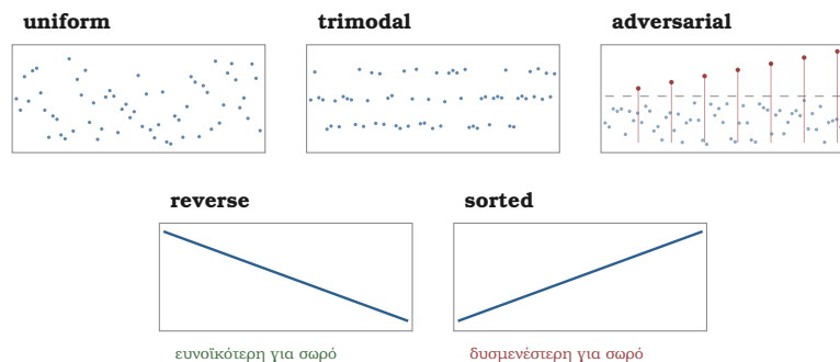
Σχήμα 3.4: Οι πέντε κατανομές εισόδου, με την τιμή κάθε στοιχείου συναρτήσεως της θέσης του στον πίνακα. Η uniform και η trimodal δεν έχουν διάταξη και διαφέρουν μόνο ως προς το ποιες τιμές εμφανίζονται· οι δύο διατεταγμένες είναι τα άκρα για την επιλογή με σωρό. Στην adversarial το σώμα των τιμών παραμένει κάτω από τη μέση τιμή του εύρους (διακεκομμένη), με μεμονωμένες αιχμές σε τακτά διαστήματα.
