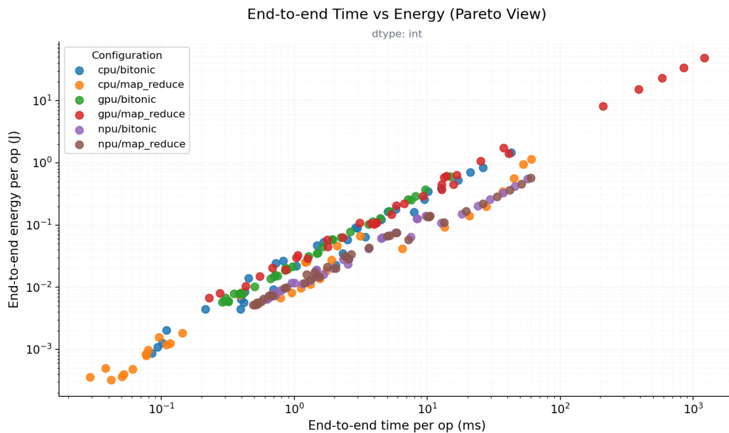
Σχήμα 7.14: Συνολικός χρόνος και συνολική ενέργεια κάθε μετρημένης περίπτωσης. Και τα δύο μεγέθη ελαχιστοποιούνται, οπότε οι προτιμότερες περιπτώσεις βρίσκονται προς την κάτω αριστερή γωνία.
