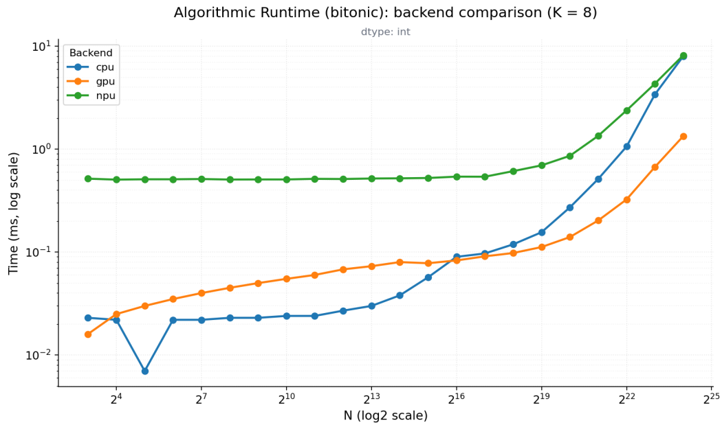
Σχήμα 7.3: Ο ίδιος αλγόριθμος στις τρεις αρχιτεκτονικές, για k ίσο με 8.
