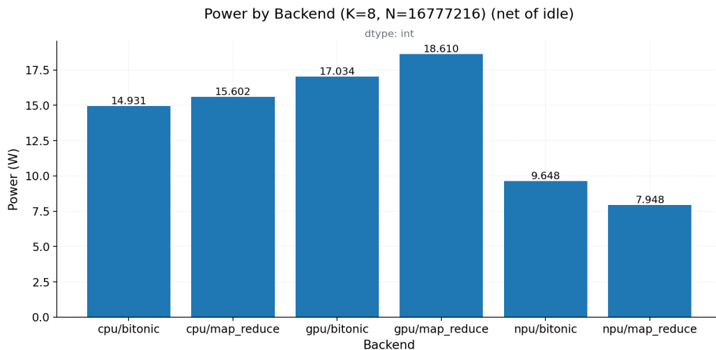
Σχήμα 7.13: Καθαρή ισχύς ανά αρχιτεκτονική και αλγόριθμο, για k ίσο με 8.
