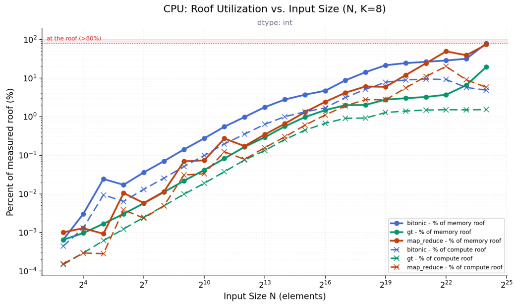
Σχήμα 7.9: Ποσοστό αξιοποίησης των δύο ταβανιών στον επεξεργαστή, για k ίσο με 8.
