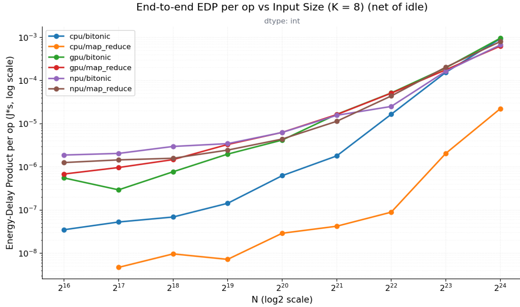
Σχήμα 7.15: Γινόμενο ενέργειας-καθυστερήσης συναρτήσει του μεγέθους εισόδου.
