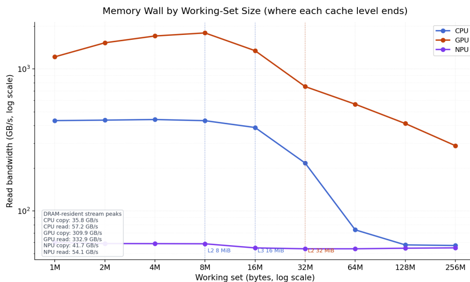
Σχήμα 7.8: Μετρημένο εύρος ζώνης ανάγνωσης συναρτήσεως του μεγέθους του συνόλου εργασίας, για τις τρεις αρχιτεκτονικές.
