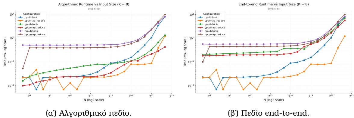
Σχήμα 7.1: Χρόνος συναρτήσει του μεγέθους εισόδου, για k ίσο με 8, στα δύο πεδία μέτρησης. Η κατάταξη των αρχιτεκτονικών ανατρέπεται πλήρως μεταξύ των δύο.
