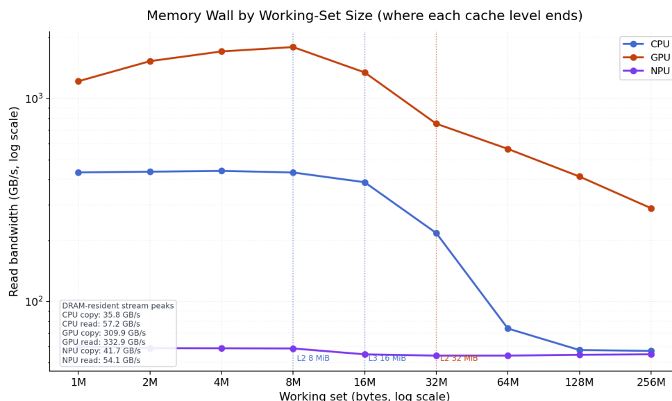
Σχήμα 7.7: Μετρημένο εύρος ζώνης ανάγνωσης συναρτήσεως του μεγέθους του συνόλου εργασίας, για τις τρεις αρχιτεκτονικές.
