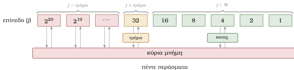
Σχήμα 4.3: Η συγχώνευση διαδοχικών επιπέδων σε ένα πέρασμα· κάθε ζεύγος βελών είναι μία ανάγνωση και μία εγγραφή ολόκληρου του πίνακα. Στο (α) κάθε επίπεδο είναι ξεχωριστό πέρασμα προς τη μνήμη· στο (β) τα επίπεδα ομαδοποιούνται κατά απόσταση j και μόνο η τελευταία ομάδα διατηρεί ξεχωριστό πέρασμα. Οι αριθμοί του σχήματος είναι ενδεικτικοί.
