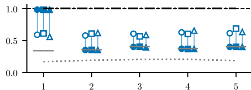
(d) r8 / r10 natural KL
