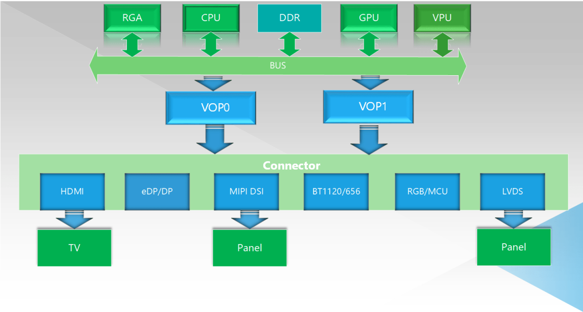
VOP 1.0 显示子系统架构
