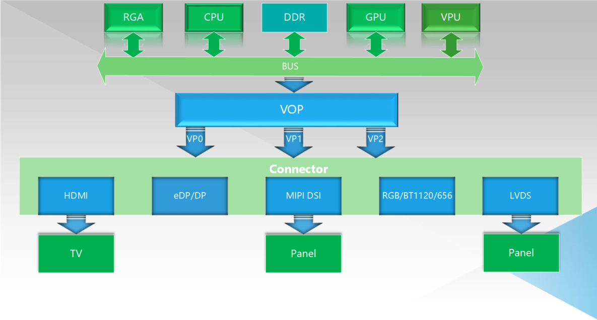
VOP 2.0 显示子系统架构
