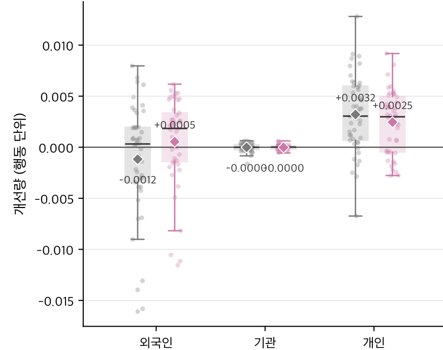
C. MAE 감소
