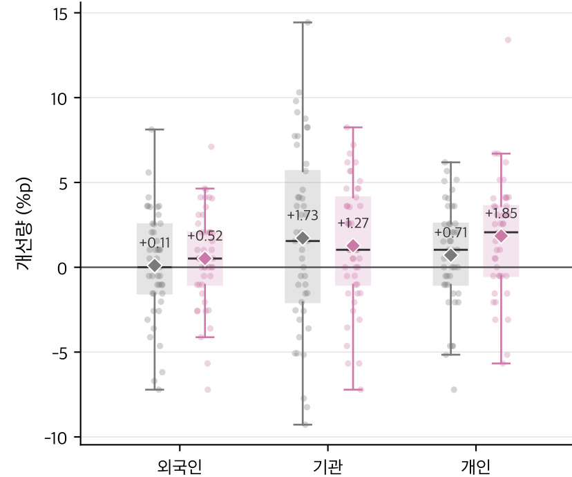
A. 방향 정확도
