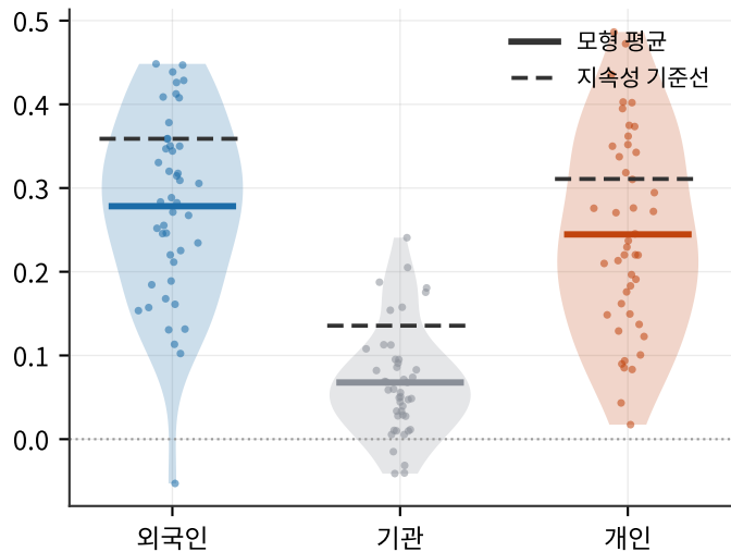
예측-실제 상관계수
