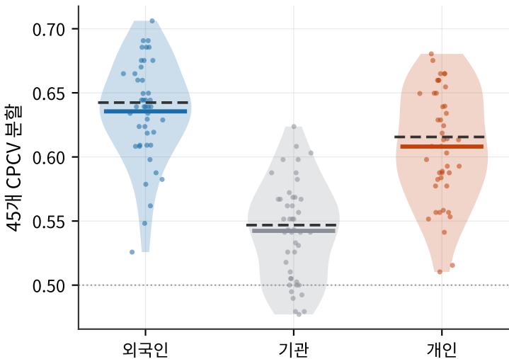
방향 정확도
