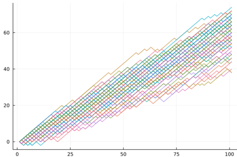
Рис. 2.2: Несимметричное случайное блуждание
