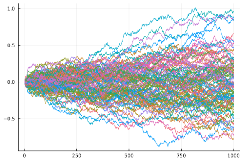
Рис. 3.1: Винеровский процесс
