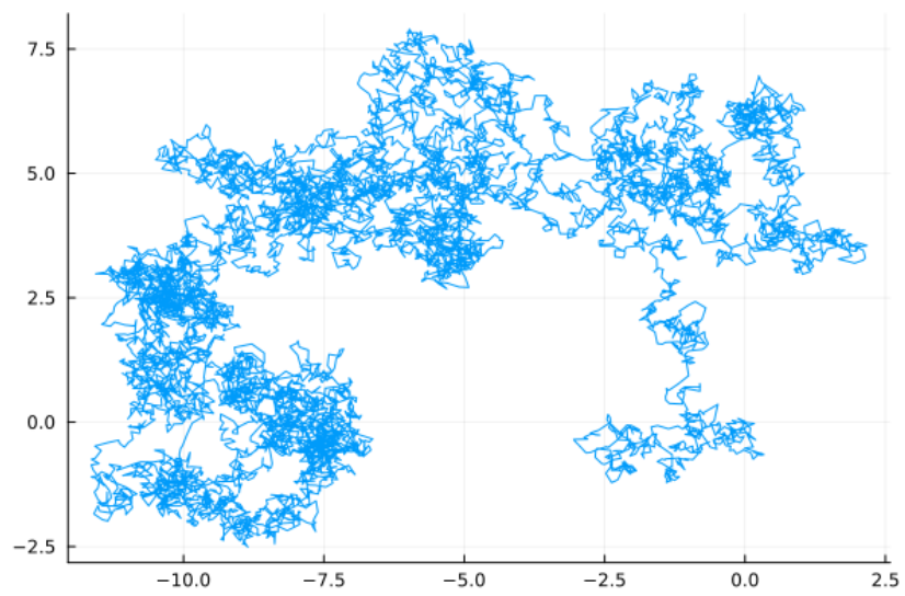
Рис. 4.2: Движение броуновской частицы. 1000 шагов
