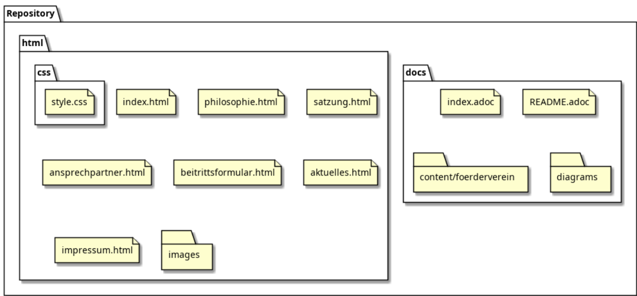
TSV Rudow Foerderverein - Project Structure
