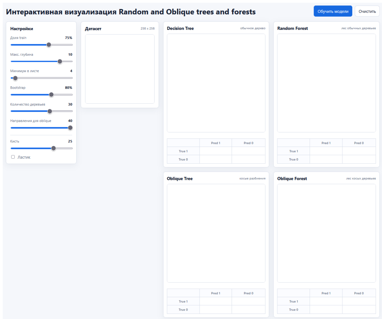
Рис. 1: Главный экран приложения: слева настройки, по центру холст, справа карточки с ответами моделей.
