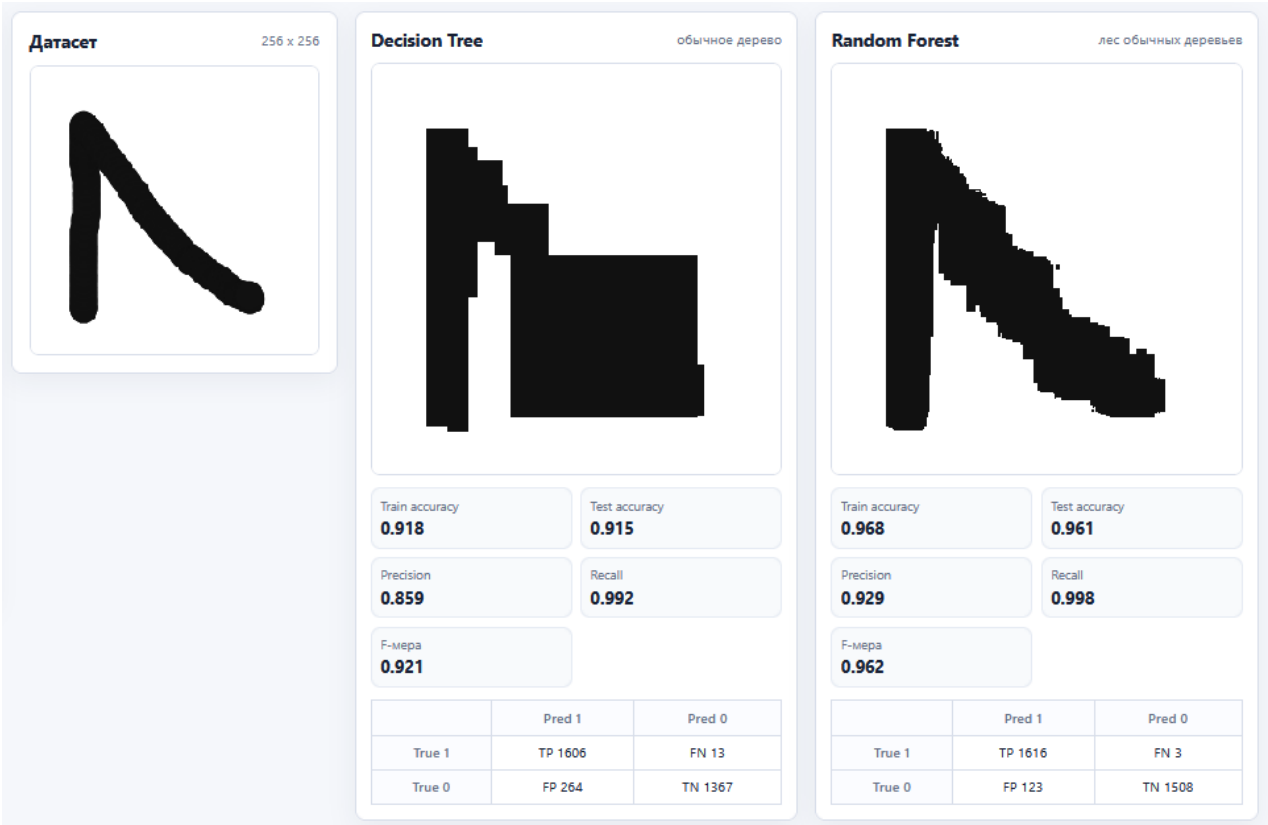
Рис. 3: Ответ случайного леса: много деревьев сглаживают ошибки друг друга.
