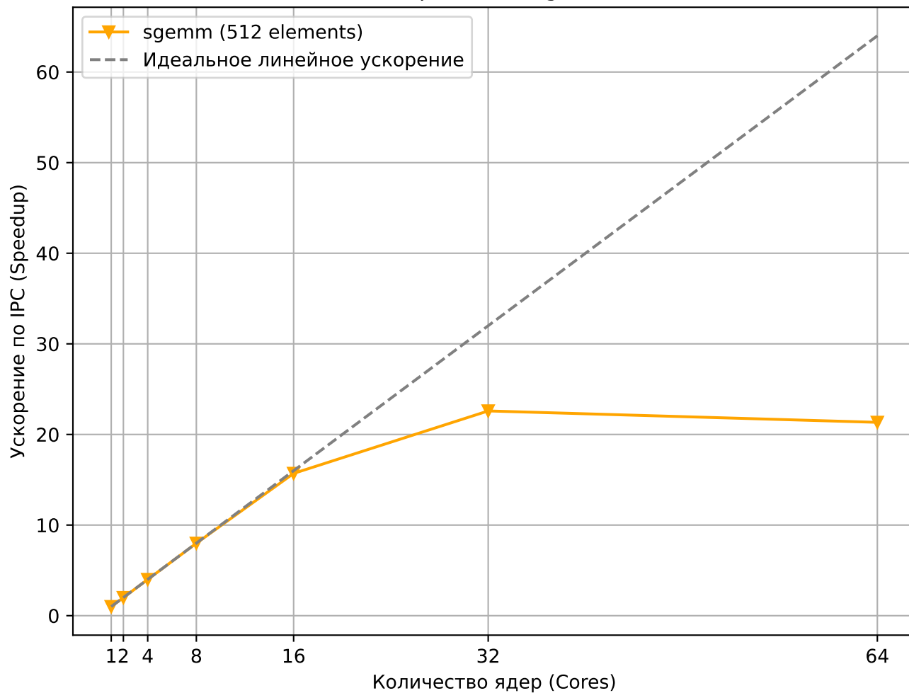
Сильное масштабирование: sgemm (512 elements)
