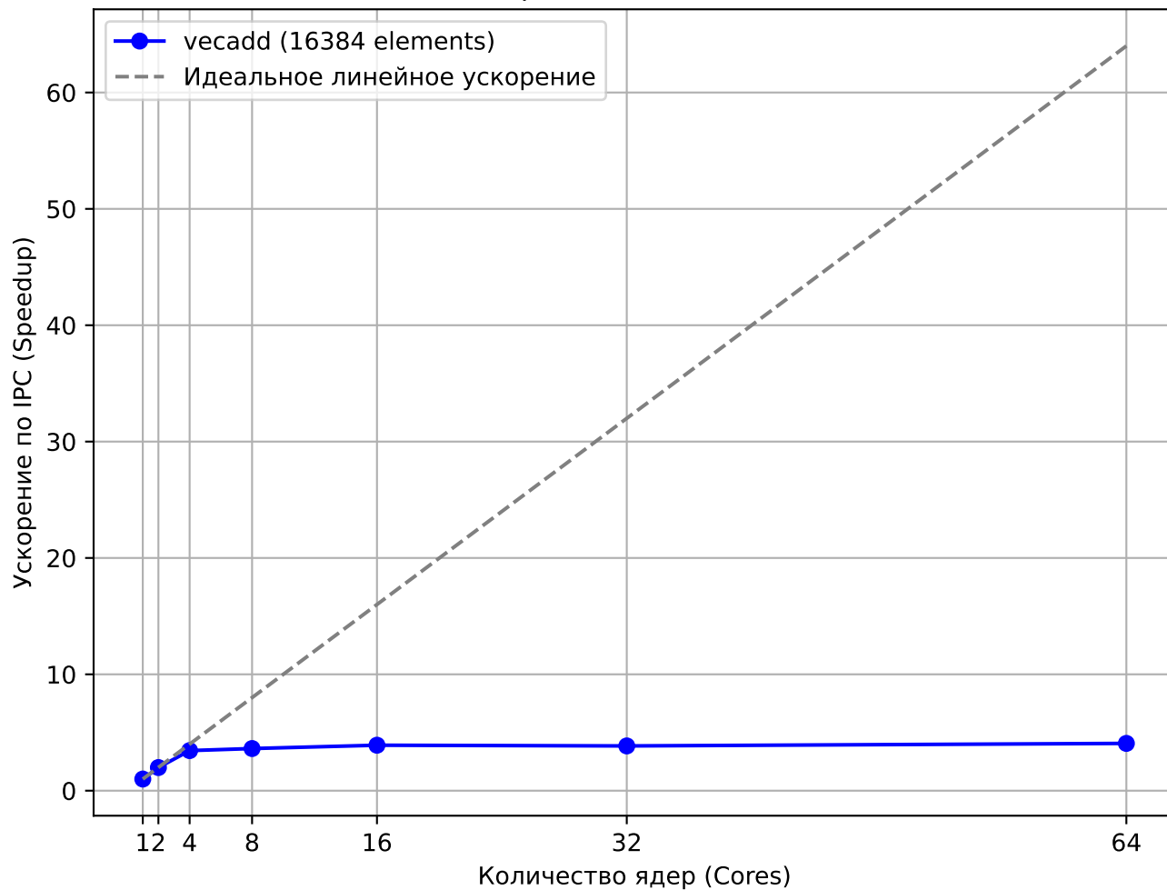
Сильное масштабирование: vecadd (16384 elements)
