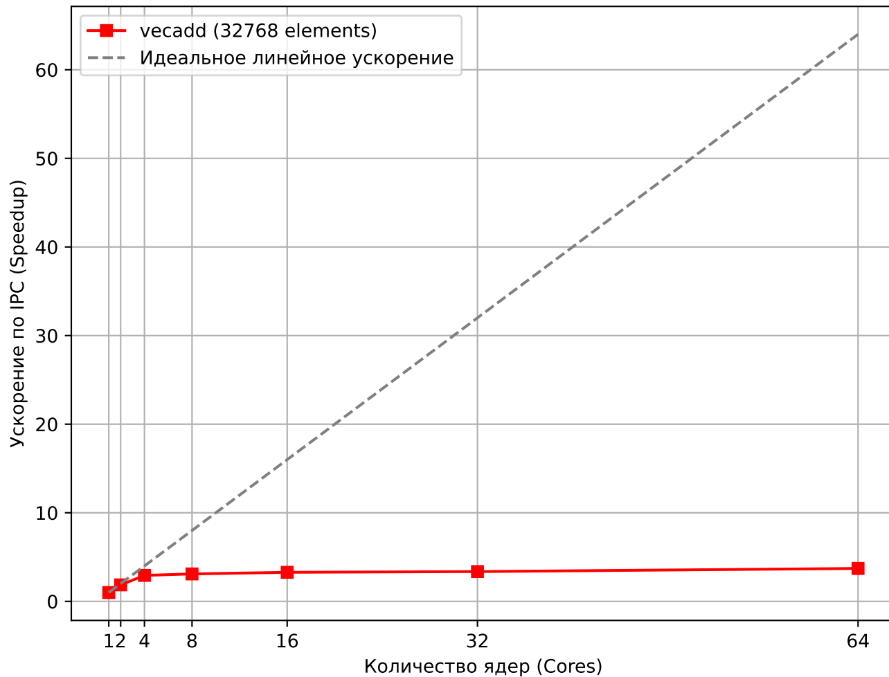
Сильное масштабирование: vecadd (32768 elements)
