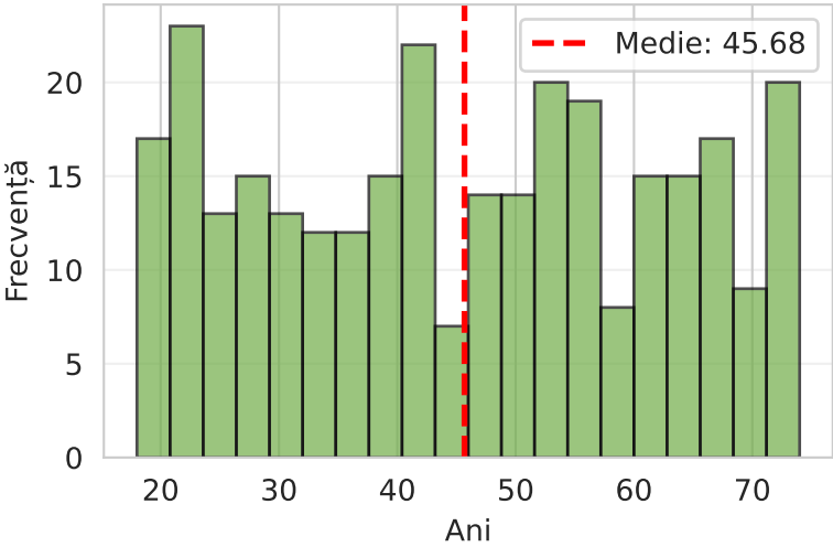
Distribuție Age
