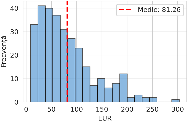
Distribuție MonthlyRevenue
