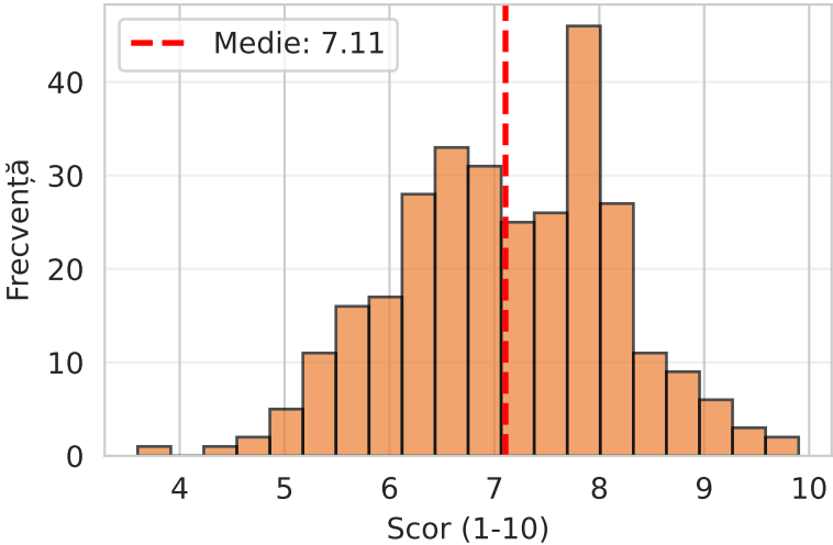
Distribuție SatisfactionScore
