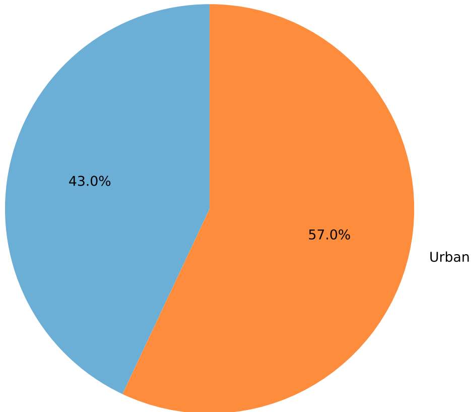
Distributia esantionului dupa Localitate
