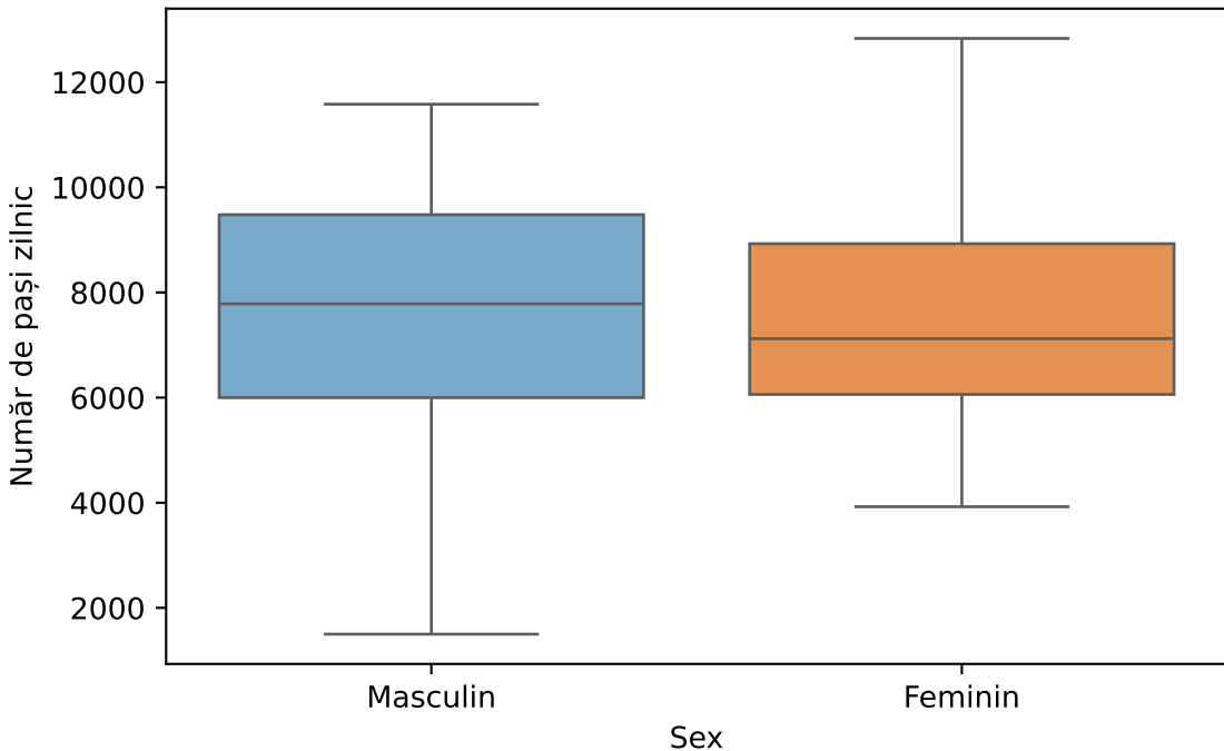
Distribuția numărului de pași zilnic după sex
