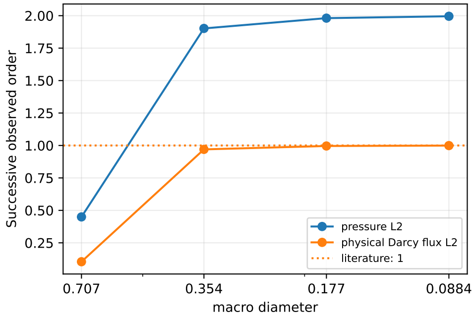
MshHO
