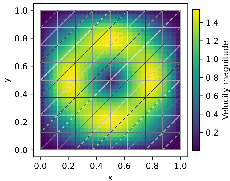
MHM: n=8 , r=4
