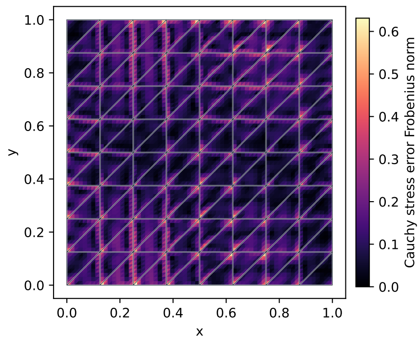
Primal MHM: n=8
