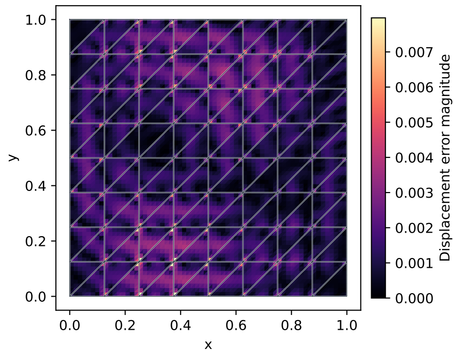
Primal MHM: n=8
