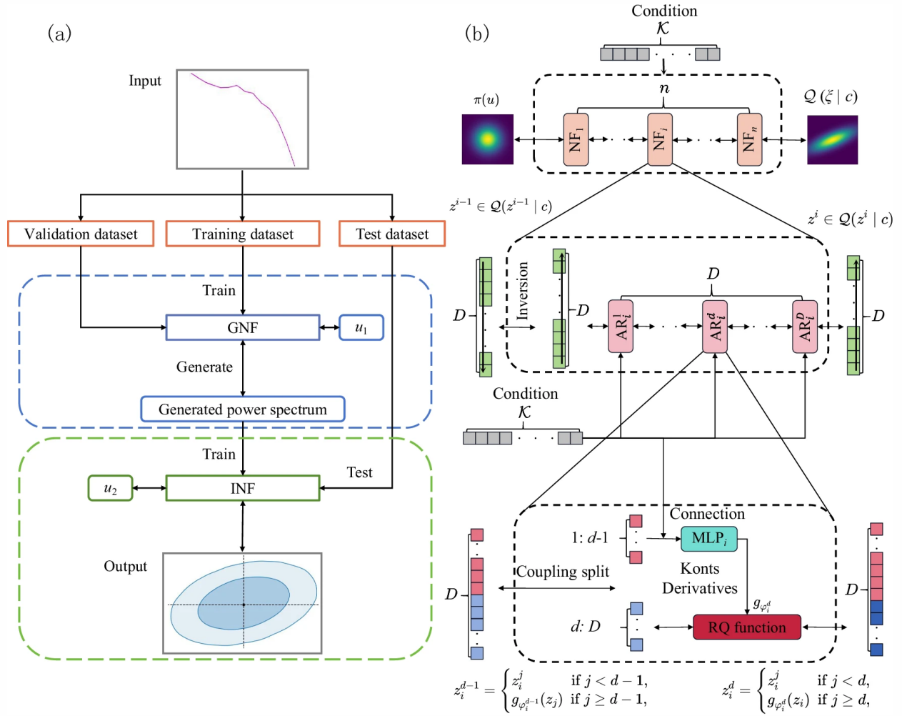
图 11.2: 21cm 森林参数推断中的双流归一化流框架。左图展示从输入功率谱划分训练集、验证集和测试集，并先训练生成归一化流（GNF）扩充模拟样本，再训练推断归一化流（INF）获得参数后验的流程；右图展示条件归一化流及自回归有理二次样条变换模块的结构。该图说明 SBI 方法在“昂贵模拟器 + 有限训练样本 + 非高斯后验”问题中的可迁移性。图引自 Sun 等 [33] 的 Figure 2。
