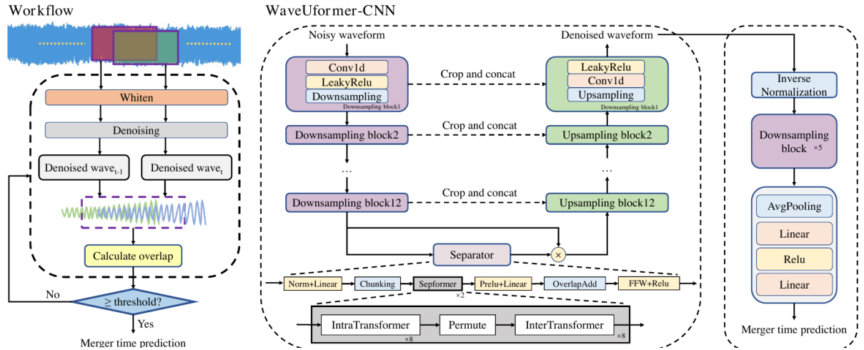
图 7.2: 长时旋近信号去噪与并合时刻预测的整体流程和 WaveUformer-CNN 架构。左侧展示滑动时间窗数据经白化和去噪后, 通过相邻窗口去噪波形的重叠度判断是否出现可用信号, 并在超过阈值后进入并合时刻预测; 右侧展示用于去噪的 WaveUformer 结构与用于并合时刻预测的 CNN 后端。图据 Xu 等 [28] 的 Figure 1 裁切引入。
