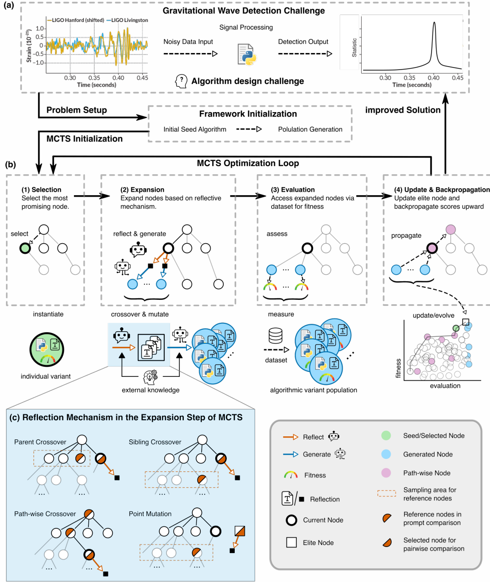
图 8.1: Evo-MCTS 框架总体流程。框架以候选引力波检测程序为搜索对象，利用 LLM 生成和反思候选代码，以 MCTS 树组织探索历史，并通过父节点交叉、兄弟节点交叉、路径级交叉和点突变等操作产生新算法；每个候选解通过 MLGWSC-1 真实噪声基准上的适应度评估获得反馈。图引自 Wang 和 Zeng [30] 的 Figure 1。
