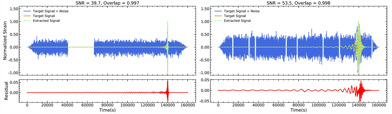
图 7.3: 深度学习模型在空间探测器非稳态噪声条件下的信号提取示例。蓝色曲线为含噪目标信号，橙色曲线为注入的目标信号，绿色虚线为模型提取信号，下方红色曲线为残差；图中两个测试样本分别给出较高信噪比条件下的重叠度结果，说明在数据异常和非稳态噪声存在时，鲁棒模型仍可恢复主要波形结构。图引自 Xu 等 [29] 的 Figure 5。
