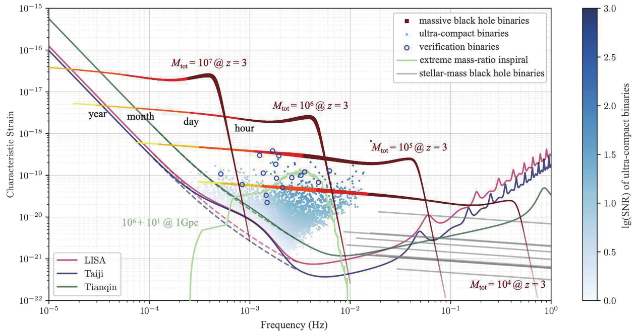
图 4.1: 空间引力波探测器 LISA、太极和天琴的设计灵敏度曲线及主要目标波源。各探测器灵敏度按等臂长近似下第一代 Michelson-AET 通道的总灵敏度给出, 纵轴为特征应变; 虚线表示仅计入探测器设备噪声, 实线表示加入银河系前景噪声后的结果。图中同时标示大质量双黑洞 (MBHB)、超致密双星 (UCB)、验证双星 (VB)、极端质量比旋入 (EMRI) 和恒星级质量双黑洞 (SBHB) 等典型源类, 用于说明空间引力波频段内多类源和前景噪声的共同存在。图引自王赫等 [12] 的 Figure 1。
