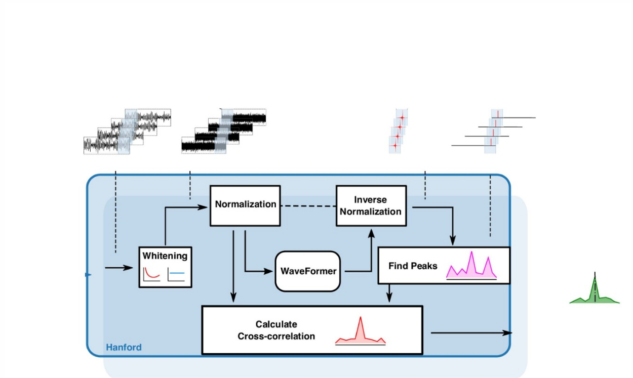
图 7.1: WaveFormer 引力波噪声抑制 workflow。LIGO 观测应变数据经过白化和归一化后输入 WaveFormer，网络输出再经反归一化、寻峰、互相关和多探测器耦合检验等后处理环节，用于验证去噪结果并服务于事件搜索；上方波形以 GW150914 为例展示输入与去噪输出的变化。图引自 Wang 等 [27] 的 Figure 1。
