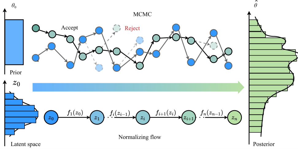
图 6.1: 传统 MCMC 采样与归一化流后验近似的流程对比。上半部分展示 Metropolis–Hastings 算法从初始参数 \theta_0 出发, 经候选采样、接受/拒绝和链式更新逐步收敛到后验样本; 下半部分展示归一化流从标准正态潜变量 z_0 出发, 通过多层可逆映射生成目标后验样本。该图直观说明了引力波参数估计中从“逐事件迭代采样”向“离线训练、在线快速生成”的方法转变。图引自 Zhao 等 [94] 的 Figure 7。
