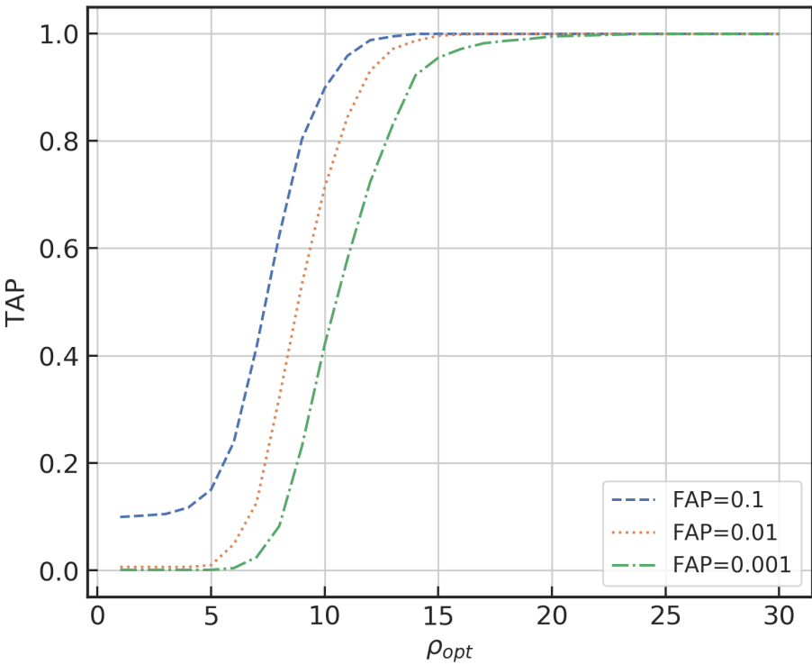
图 5.2: MF-CNN 在真实 LIGO O1 背景噪声注入测试中的识别效率随最优匹配滤波信噪比 \rho_{opt} 的变化。纵轴为正报几率 (TAP)，三条曲线对应固定误报几率 FAP = 0.1, 0.01, 0.001 的情形；在更严格的误报控制下，达到同等 TAP 所需的 \rho_{opt} 更高。图引自 iPhysResearch 的 MF-CNN 章节，相关实验设置见 Wang 等人 [20, 79]。
