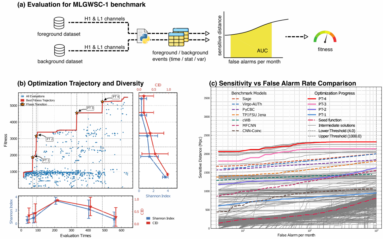
图 8.3: Evo-MCTS 的优化动力学与 MLGWSC-1 基准验证。图中展示了框架如何接入标准化适应度评估、多个独立搜索运行中的阶梯式性能跃迁，以及 PT-1 至 PT-4 相对多种基线方法的敏感距离曲线改进。图引自 Wang 和 Zeng [30] 的 Figure 3。
