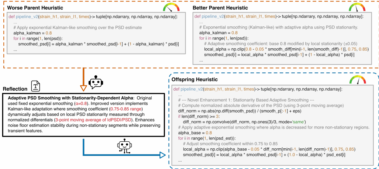
图 8.2: Evo-MCTS 中的树结构进化操作示例。图中展示了从已有候选程序出发，通过局部参数调整、领域知识约束和 LLM 反思生成新候选的过程；候选节点携带适应度反馈，使搜索既保留高分路径，又能沿低访问分支探索潜在改进。图引自 Wang 和 Zeng [30] 的 Figure 2。
