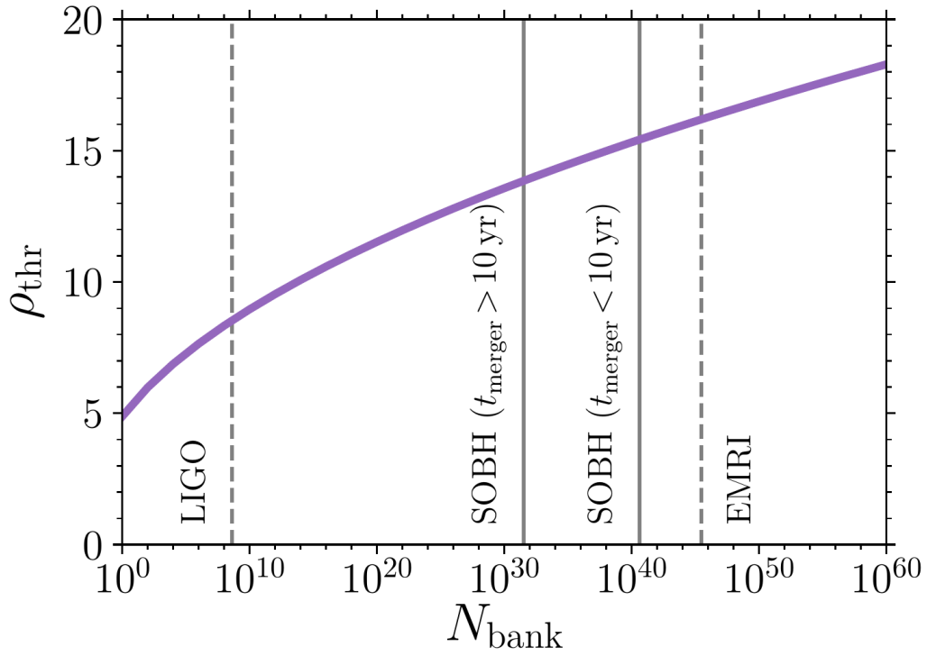
图 4.2: 模板库规模对引力波搜索阈值 SNR 的影响。横轴为有效模板数 N_{\text{bank}} , 纵轴为在固定误报控制下所需的阈值 SNR; 图中竖线比较了 LIGO/Virgo 双黑洞搜索、LISA 中恒星质量双黑洞 (SOBH) 快慢啁啾情形以及 EMRI 搜索的典型模板库规模。该图表明, 空间探测器中的长寿命信号会显著放大模板库规模和试验因子, 使可探测阈值从地面探测器常见的 \rho \sim 8 提高到 \rho_{\text{thr}} \sim 14\text{--}15 , 甚至更高。图引自 Moore、Gerosa 与 Klein [58] 的 Figure 1。
