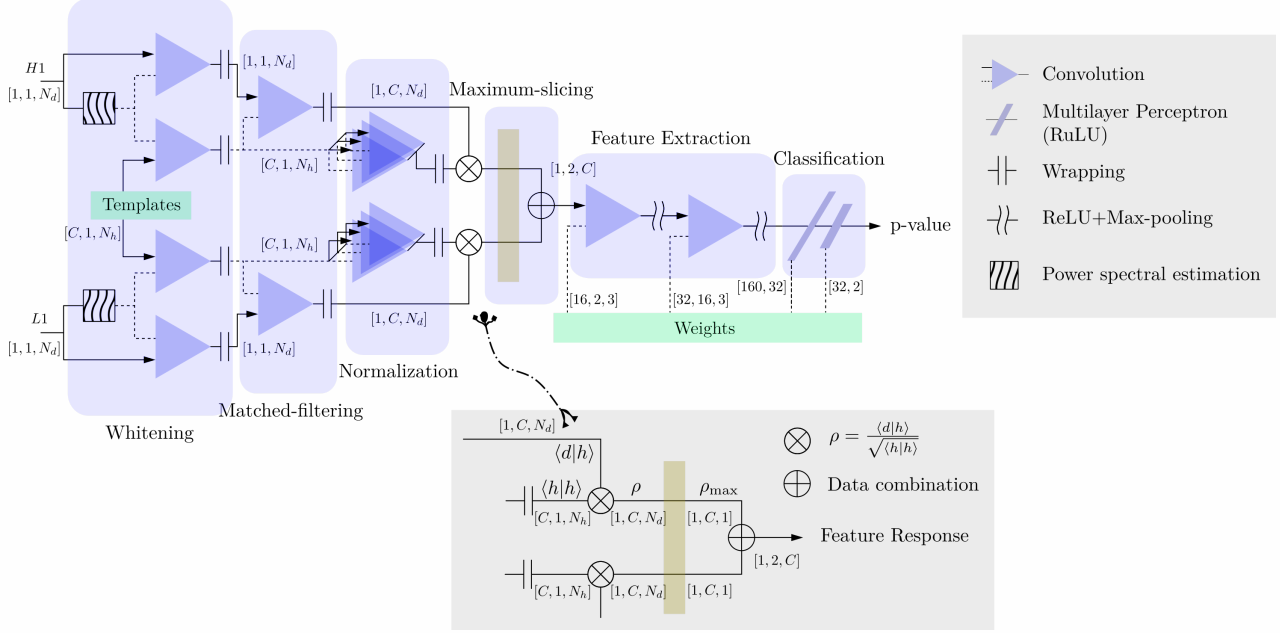
图 5.1: MF-CNN 网络架构示意图。输入的双探测器时域数据先进入白化、匹配滤波和归一化卷积单元，得到每个模板与每个探测器通道的匹配滤波响应；随后通过最大化切片提取特征响应 \rho_m[1, 2, C] ，并交由后续卷积网络和分类层输出候选信号概率。该图引自 iPhysResearch 的 MF-CNN 章节，并对应 Wang 等人 [20, 79] 的网络构造。
