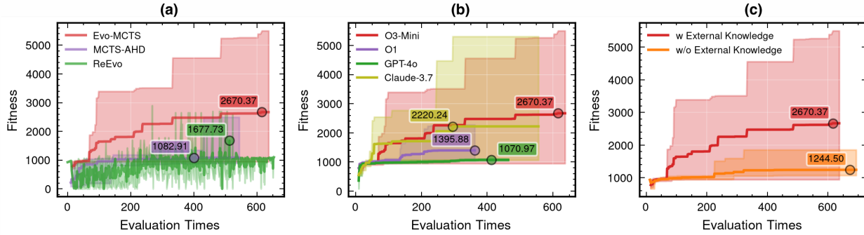
图 8.5: Evo-MCTS 在不同设计选择下的适应度演化。左图比较 Evo-MCTS、MCTS-AHD 和 ReEvo，显示树搜索与进化操作结合带来的优势；中图比较不同基础 LLM 的搜索表现；右图显示外部领域知识注入对搜索效率和最终适应度的影响。图引自 Wang 和 Zeng [30] 的 Figure 6。
