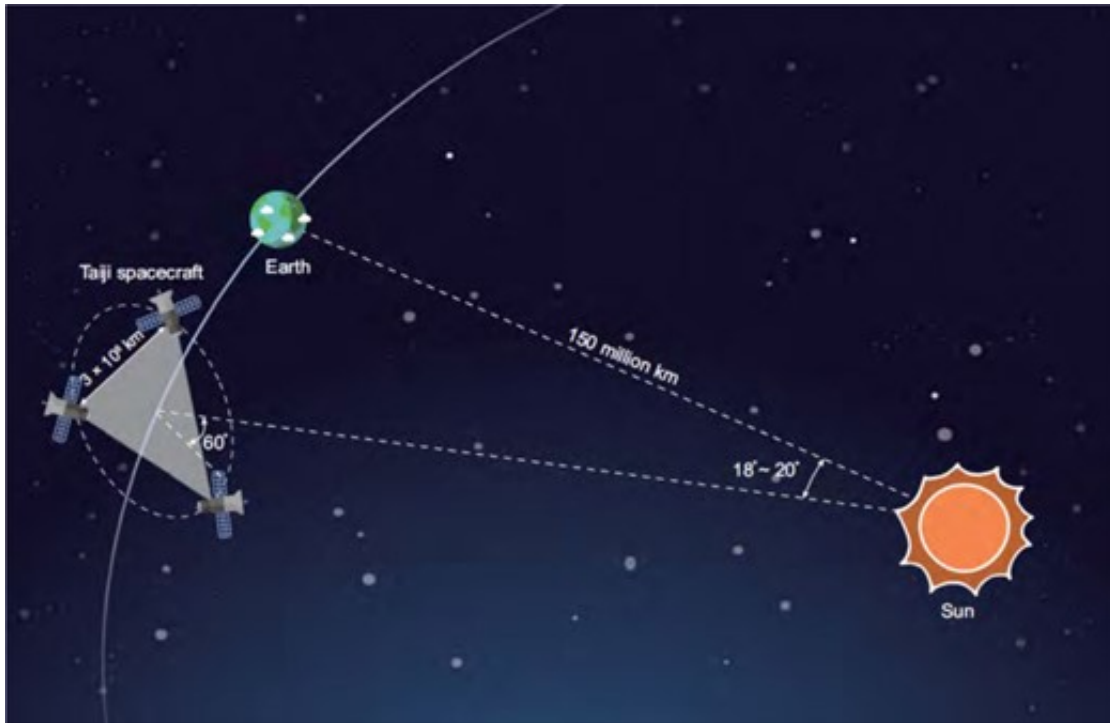
图 10.1: 太极 (Taiji) 空间引力波探测器星座示意图。太极三颗航天器构成臂长约 3 \times 10^6 km 的近似等边三角形星座, 星座中心沿日心轨道运行, 并与地球保持约 18^\circ - 20^\circ 的角距离。该轨道构型使太极在毫赫兹频段获得长期稳定的空间干涉基线, 也为与 LISA 等日心轨道任务开展联合观测提供了方向图互补性。图片引自 Luo 等 [122] 的 Figure 1。
