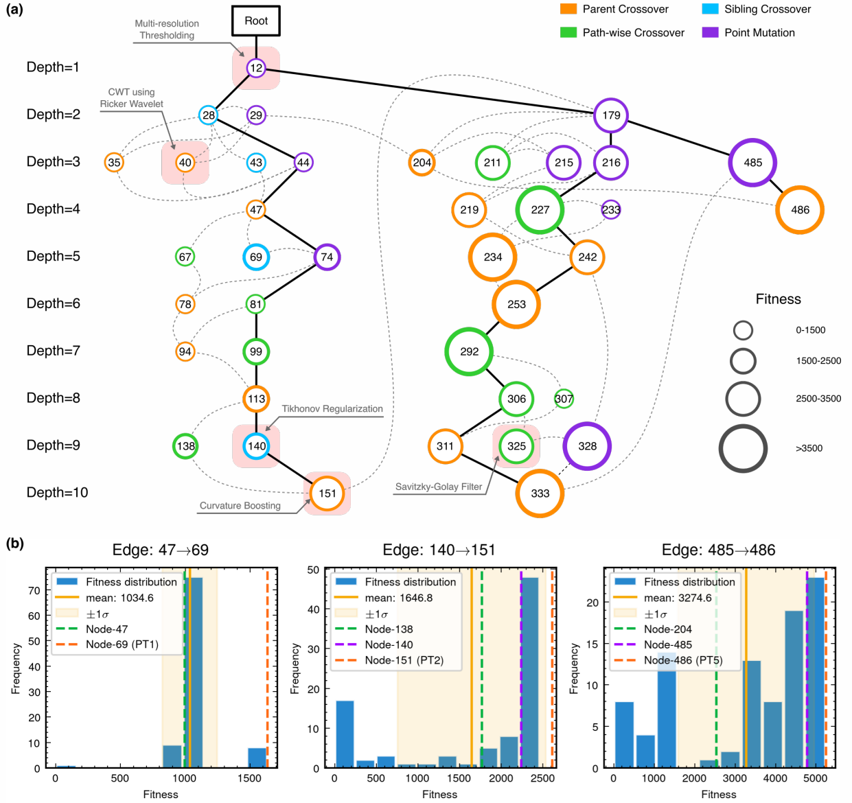
图 8.4: Evo-MCTS 搜索树中的关键算法节点与可重复性分析。上半部分展示节点编号、边关系、节点类型和若干关键算法模块的引入位置；下半部分通过对代表性边的重复生成实验，显示部分改进在独立重演中能够稳定超过父节点，支持“可解释算法路径”并非单次偶然搜索结果。图引自 Wang 和 Zeng [30] 的 Figure 5。
