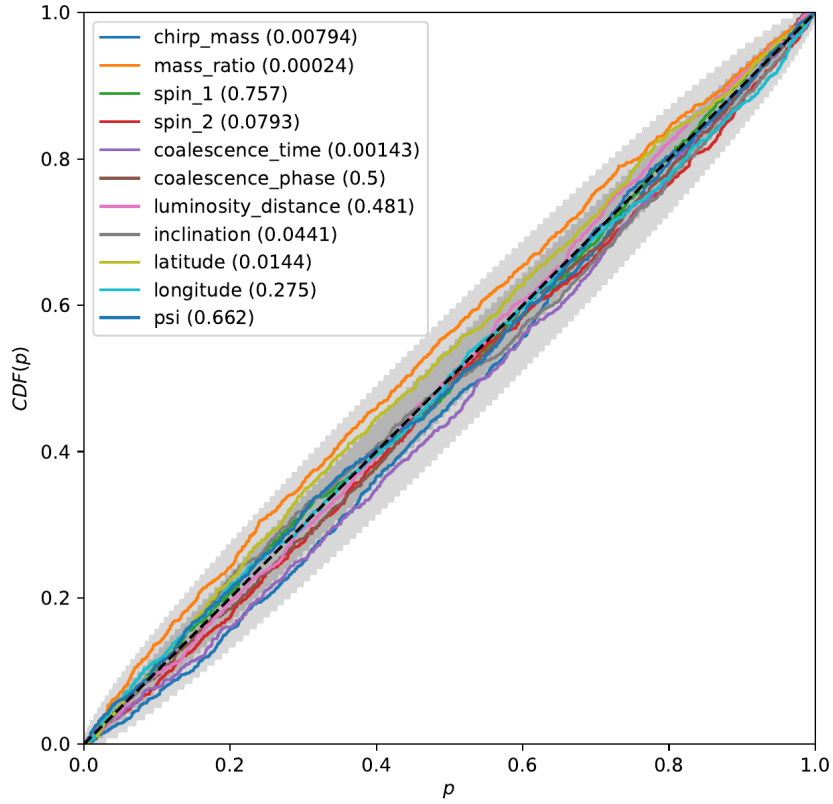
图 6.3: 太极大质量双黑洞归一化流参数估计的 P-P 图覆盖率验证。横轴为真实参数在一维边缘后验中的分位数 p ，纵轴为这些分位数的累积分布 CDF(p) ；理想校准对应角线，灰色区域表示 1\sigma 和 2\sigma 置信带。图中多条曲线对应啁啾质量、质量比、自旋、并合时间、距离和天空位置等参数，图例括号内为 KS 检验 p 值。该图来自 Du 等 [22] 的 P-P plot。
