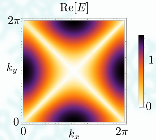
Real Fermi arcs
