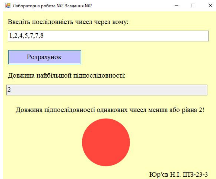
Рис. 3. Результат виконання програми
