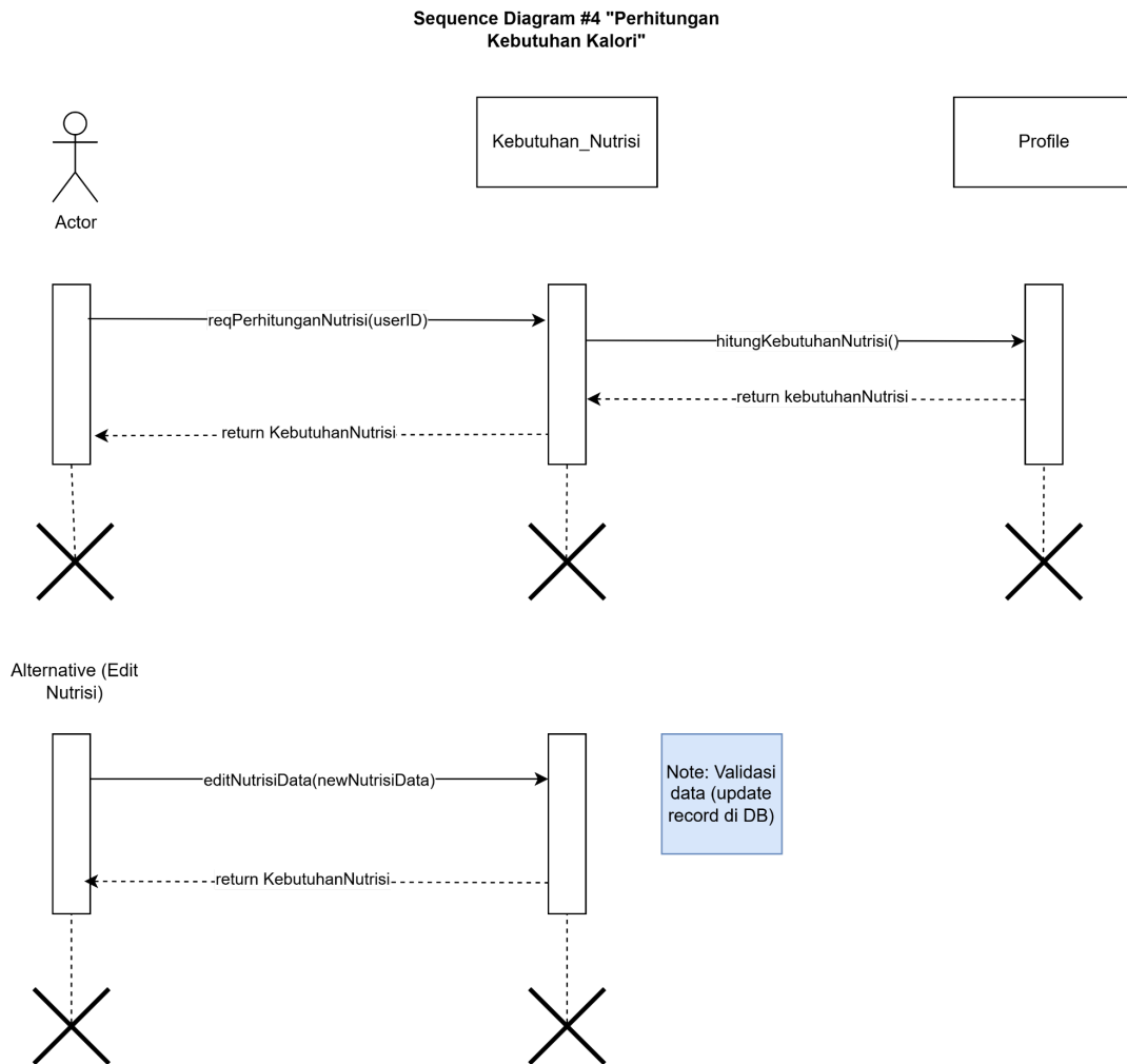
Gambar 3.1.4.4 - Perhitungan Kebutuhan Kalori
