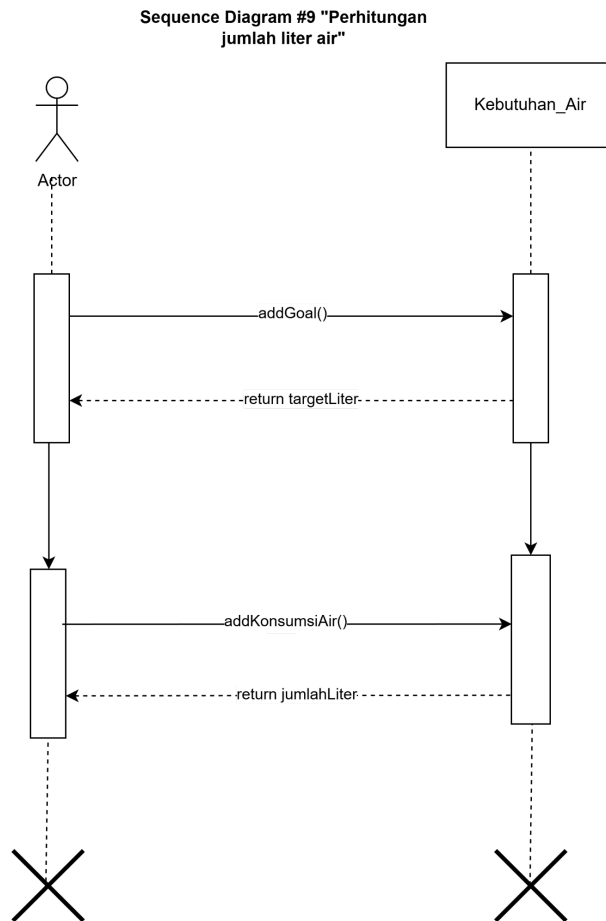
Gambar 3.1.9.4 - Perhitungan Jumlah Liter Air
