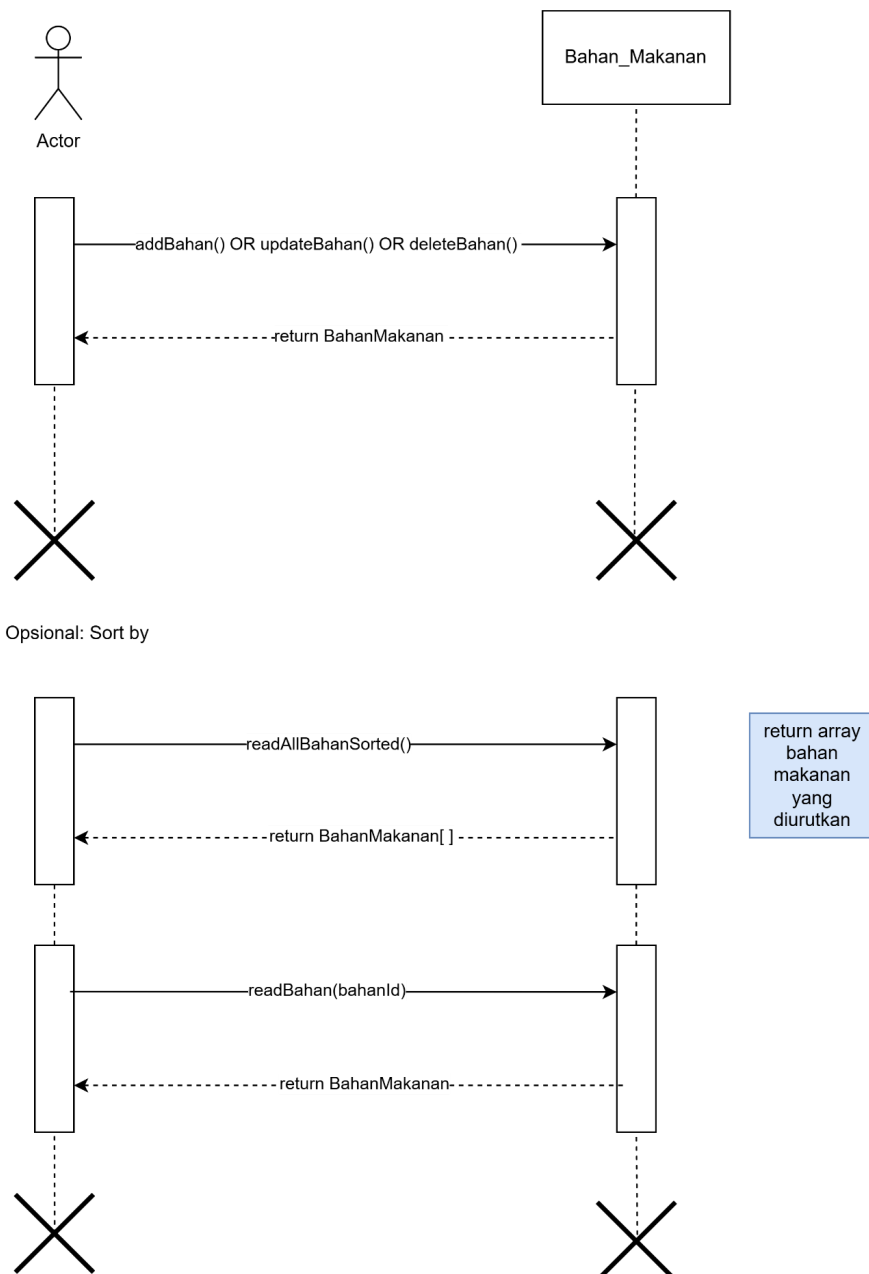
Sequence Diagram #5 "Pengelolaan Bahan Makanan"
