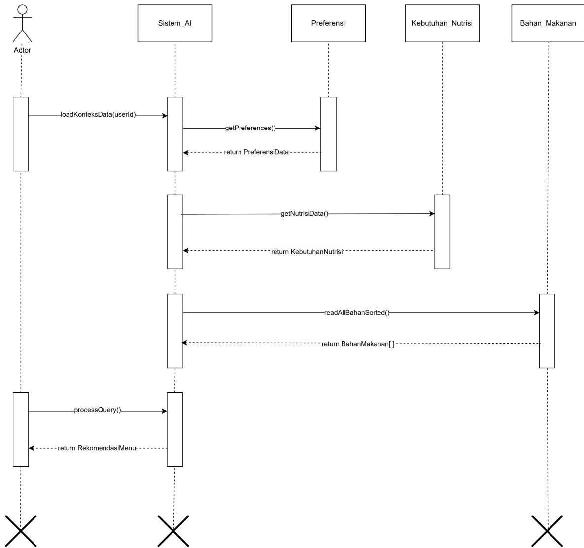
Gambar 3.1.6.4 - Pemberian Rekomendasi Makanan
