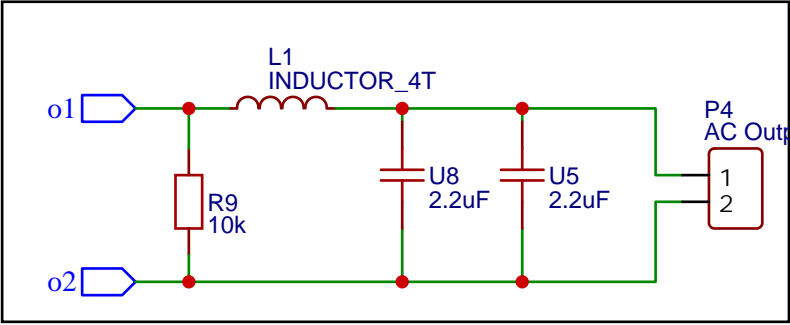
Output AC
