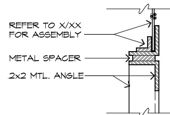
11 DETAIL SCALE: 3" = 1'-0"
