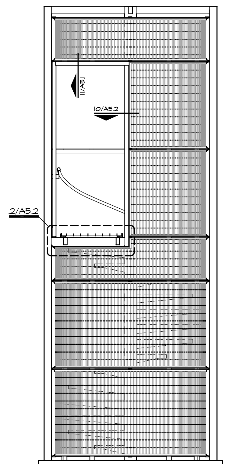
3 ELEV./SECTION SCALE: 3/8" = 1'-0"
