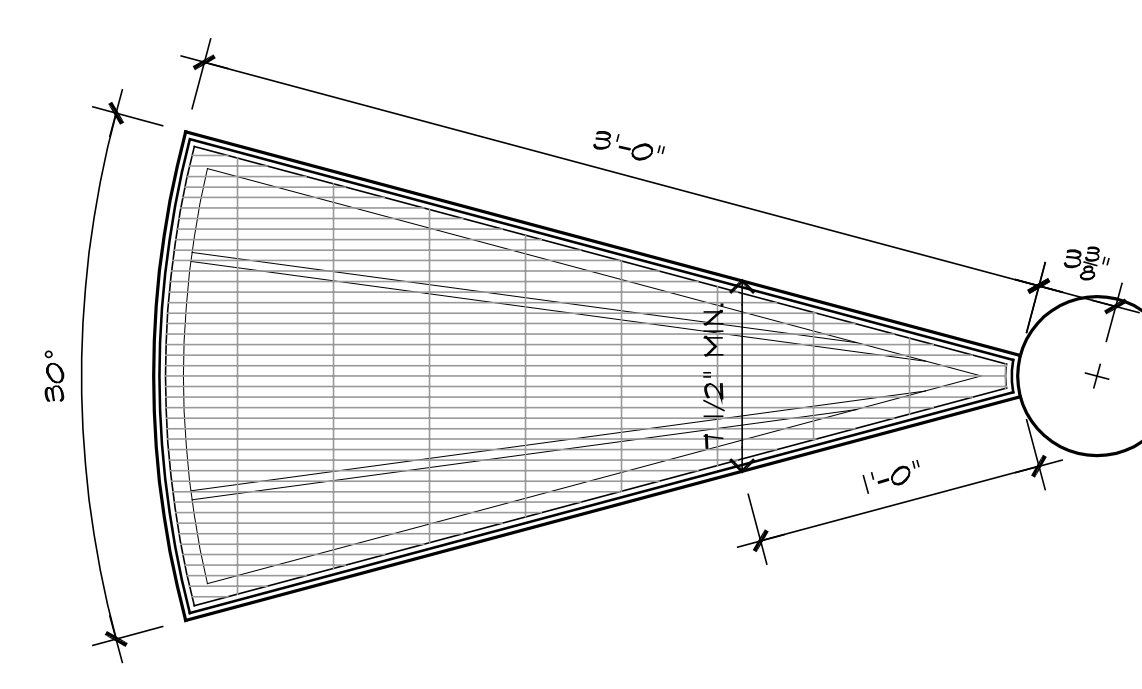
5 DETAIL SCALE: 1 1/2" = 1'-0"
