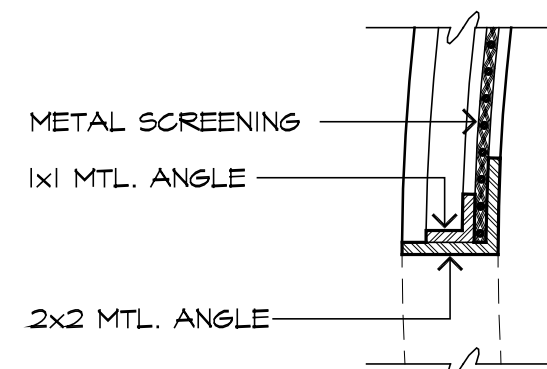
10 DETAIL SCALE: 3" = 1'-0"
