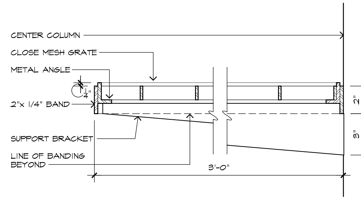
6 DETAIL SCALE: 3" = 1'-0"
