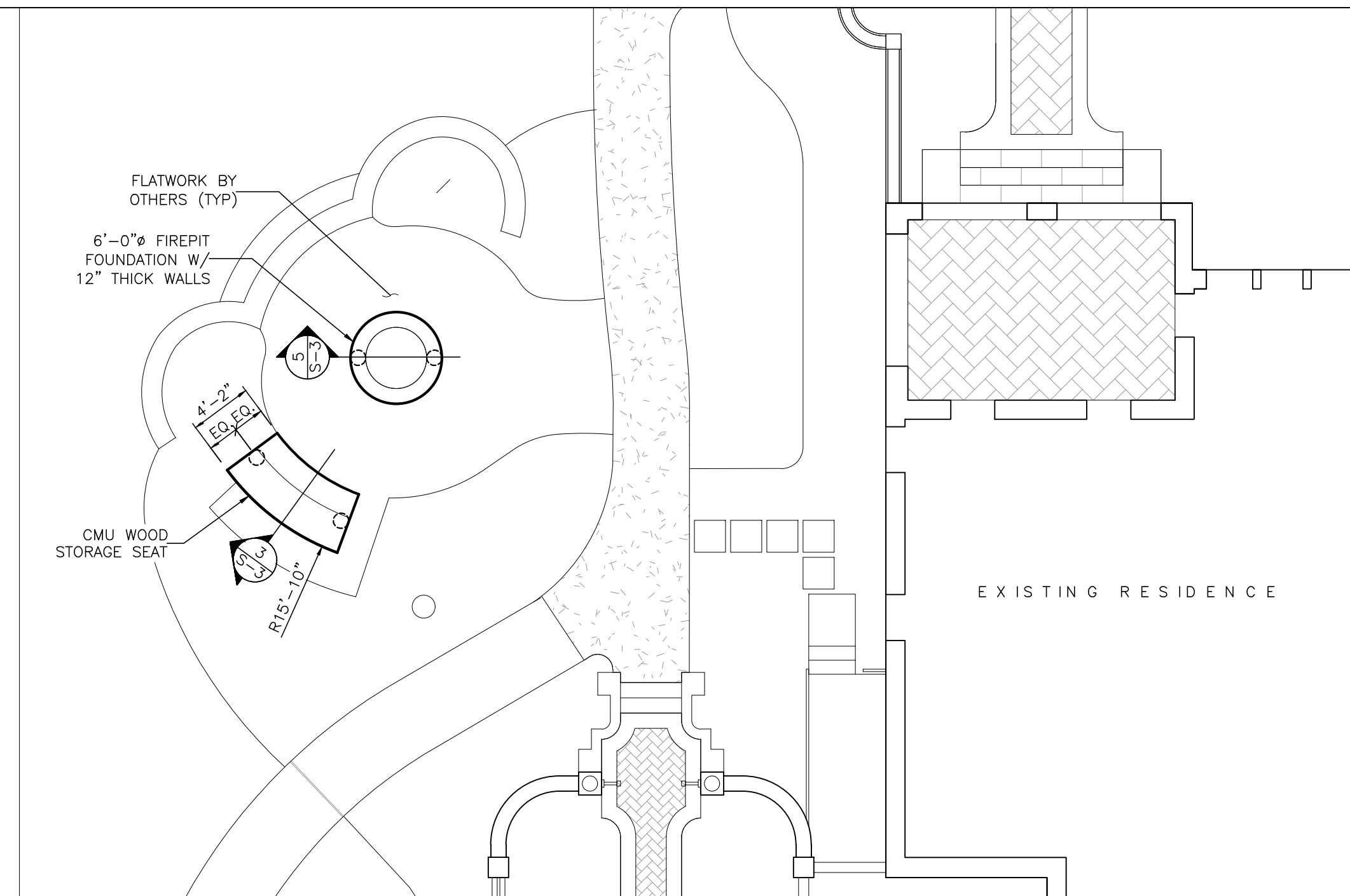
FIREPIT PLAN SCALE: 1/8" = 1'-0"
