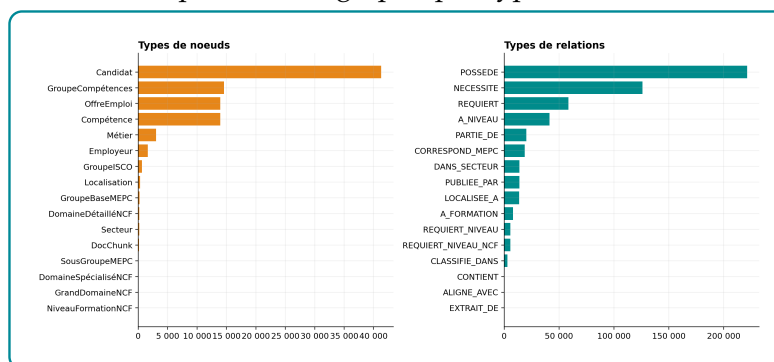
Figure A.3 – Composition du graphe par types de noeuds et relations
