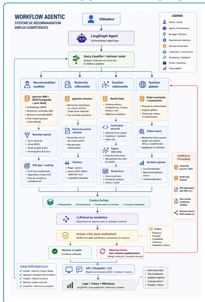
Figure 2.1 – Architecture méthodologique du workflow agentique de recommandation
