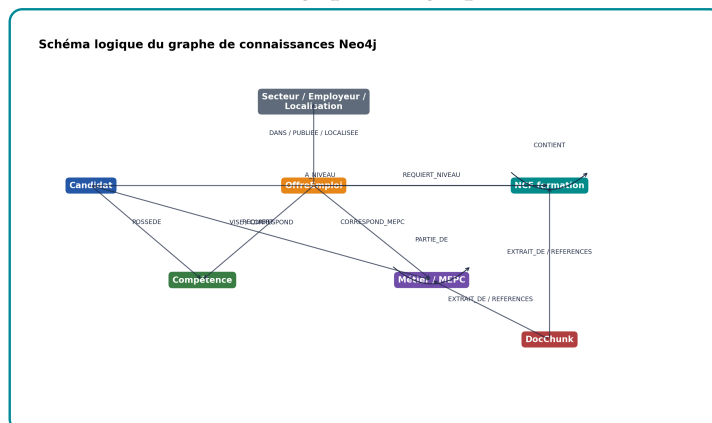
Figure 3.10 – Schéma logique du graphe de connaissances
