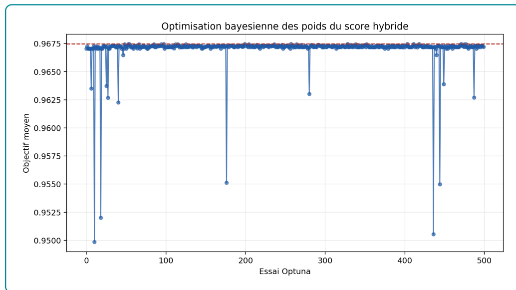
Figure 4.4 – Évolution de l'objectif NDCG@10 au cours des essais Optuna
